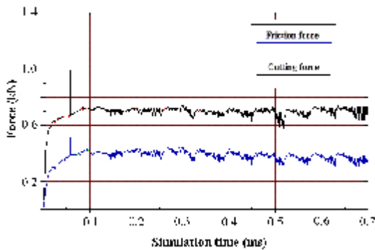
شکل ۸: نیروهای برشی در شبیه سازی با فرکانس مشرریزی متغییر.
