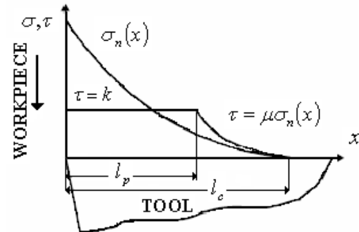
شکل ۳: تنش‌های عمودی و اصطکاک در سطح براده ابزار.
