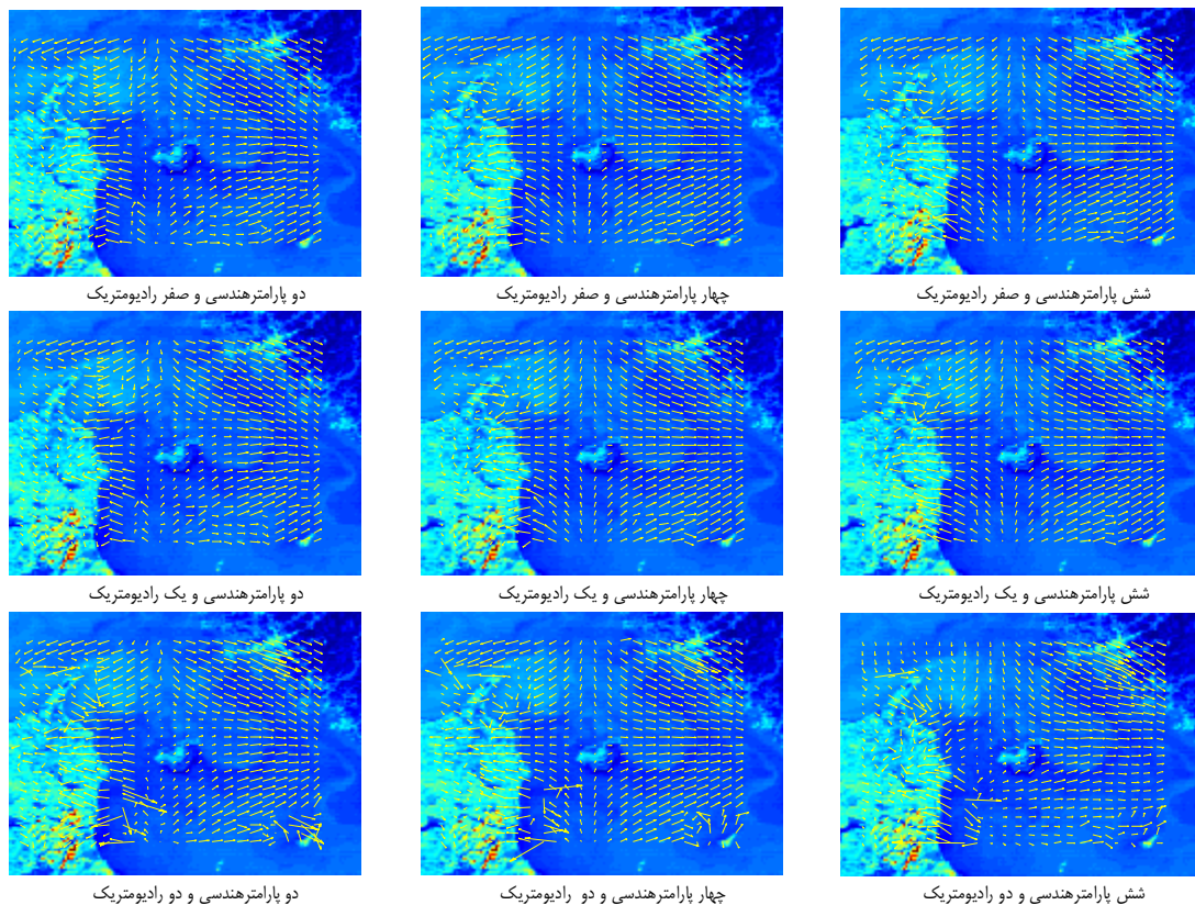
شکل ۲: جریان نوری استخراج شده در روش تناظریابی کمترین مربعات در تصویر شبیه‌سازی شده.
