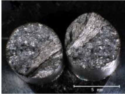
شکل ۳: سطح مقطع شکست دو نیمه یک نمونه آزمایش استحکام کششی از جنس Al-Si-Mg که دو لایه اکسید کاملاً متقارن را نشان می دهد [۸].
