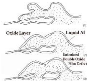
شکل ۱: نحوه ایجاد فیلم اکسید دوتایی [۲].
