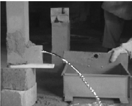
شکل ۶: آزمایش ۲، محاسبه سرعت حرکت مذاب در راهبار قبل از فیلتر توسط اندازه گیری دبی خروجی جریان.
