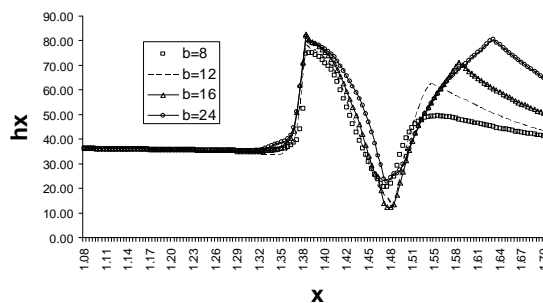
شکل ۱۶: مقایسه ضرایب انتقال حرارت بر روی صفحه تخت در جریان آشفته ( Re_x = 10^6 ) برای مانع مستطیلی با ابعاد (8mm \times bmm) در فاصله D = 4mm از صفحه تخت.
