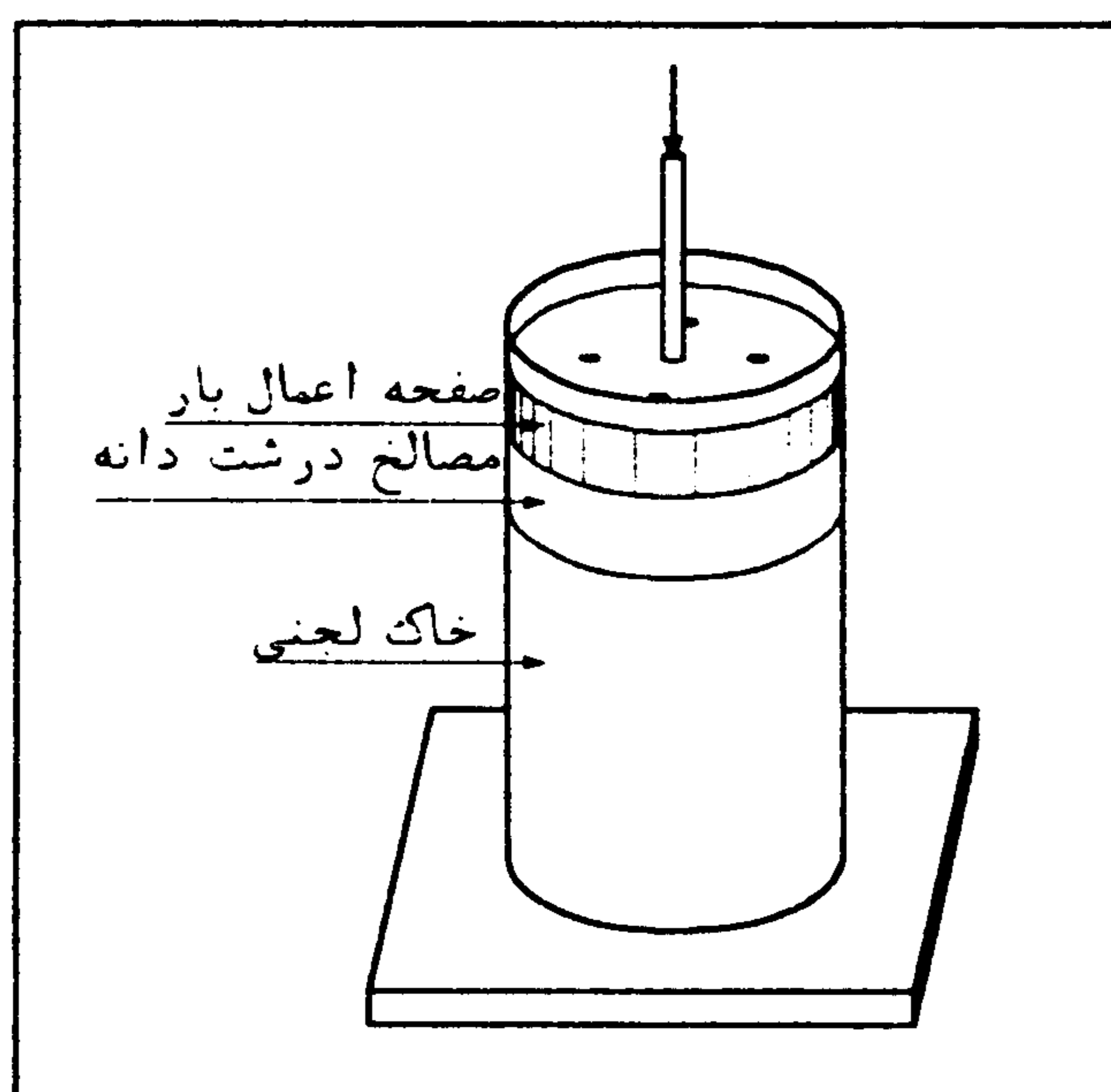
شکل ۲: چگونگی اعمال بار بر روی نمونه.
