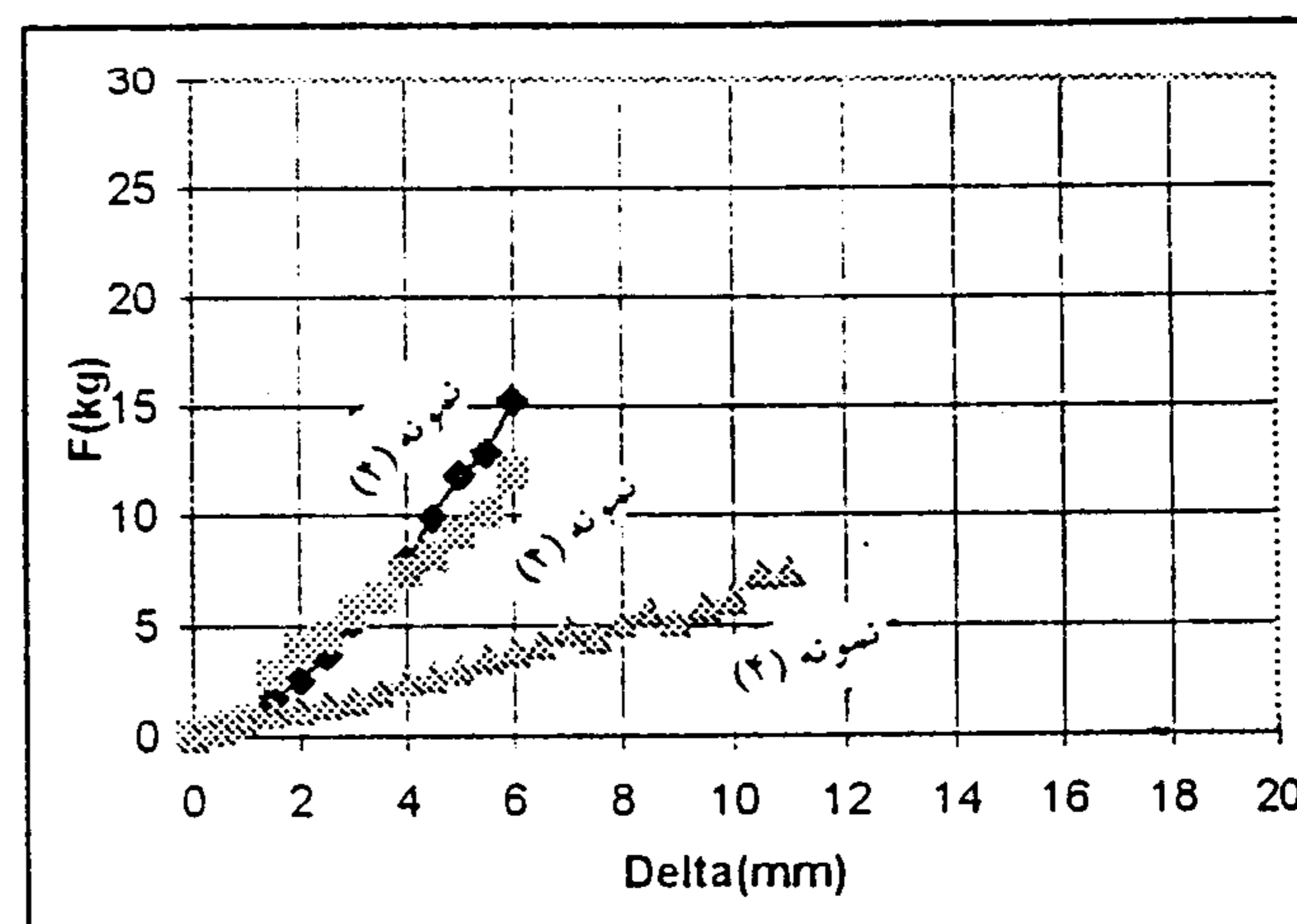
شکل ۵: بررسی تکرار پذیری آزمایش ها.
