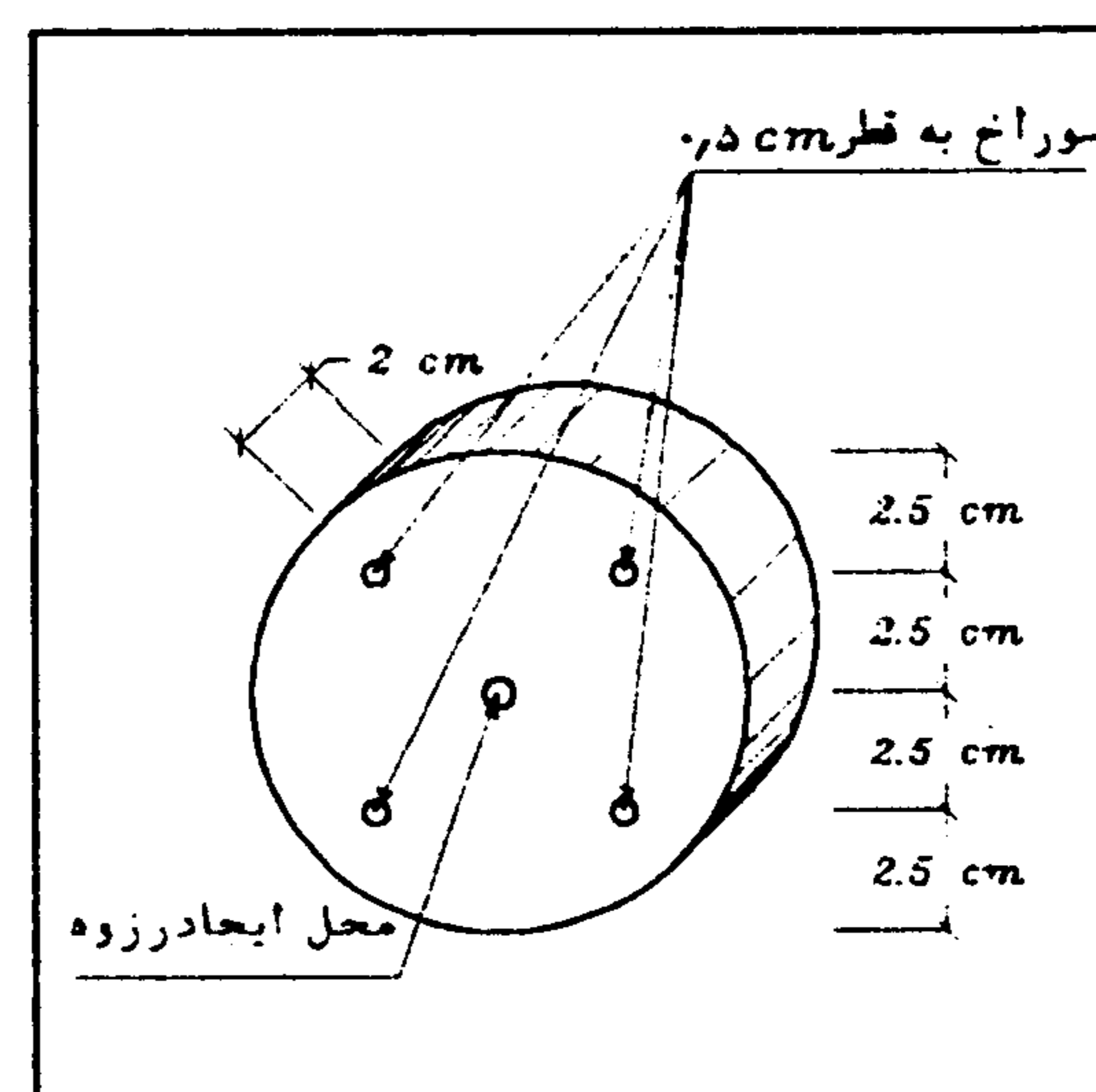
شکل ۱: صفحه اعمال بار.
