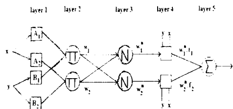
شکل ۳: یک سیستم فازی نوع سوگنو به همراه شبکه ANFIS معادلش.
