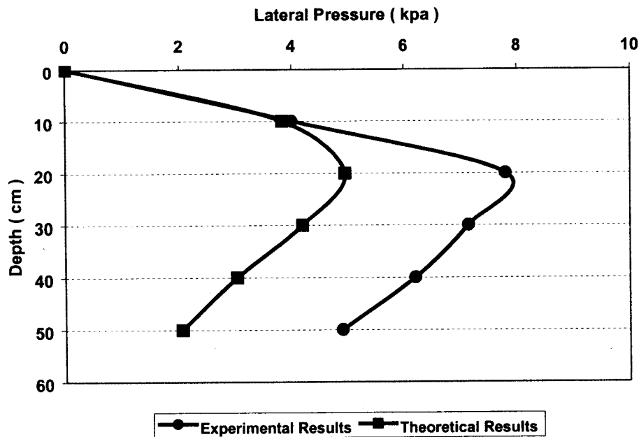
شکل ۶: نمودار مقایسه تغییرات رانش خاک حاصل از آزمایش با رابطه تنوری تحت اثر سربار استاتیکی.
