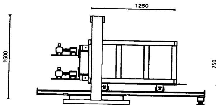
شکل ۲: مقطع طولی مخزن خاک به همراه قاب اصلی و سیستم محرک دیوار حائل (ابعاد بر حسب میلی‌متر).
