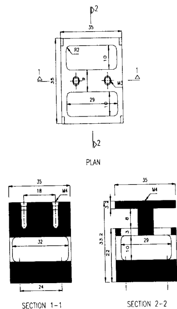
شکل ۵: تصاویر ترانسدیوسرهای مرکب (دو منظوره) جهت اندازه گیری همزمان فشار و برش در روی مدل دیوار حائل (ابعاد بر حسب میلیمتر).
