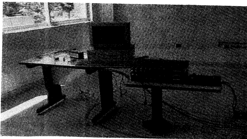
شکل ۴: تصویری از سیستم قرائت وضبط داده ها شامل دیتا لاگر، کامپیوتر، ترانسدیوسرهای تغییر مکان، نیرو و تنش.
