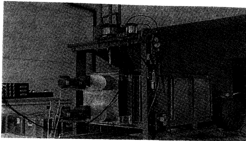
شکل ۳: تصویری از سیستم بارگذاری طراحی شده جهت اعمال سربارهای استاتیکی و سیکلی به خاک پشت دیوار حائل.
