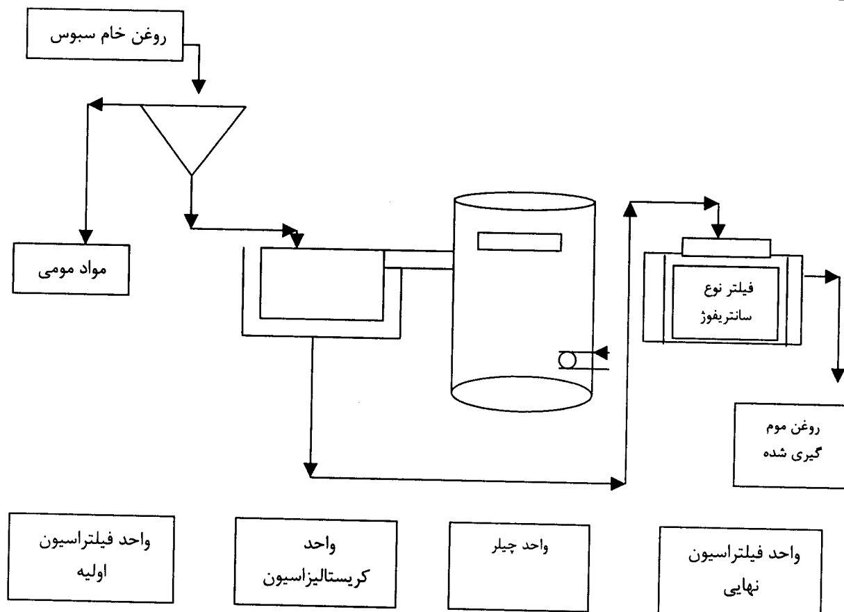
شکل ۱: نمای فرآیند واحد موم گیری از روغن سبوس برنج.
