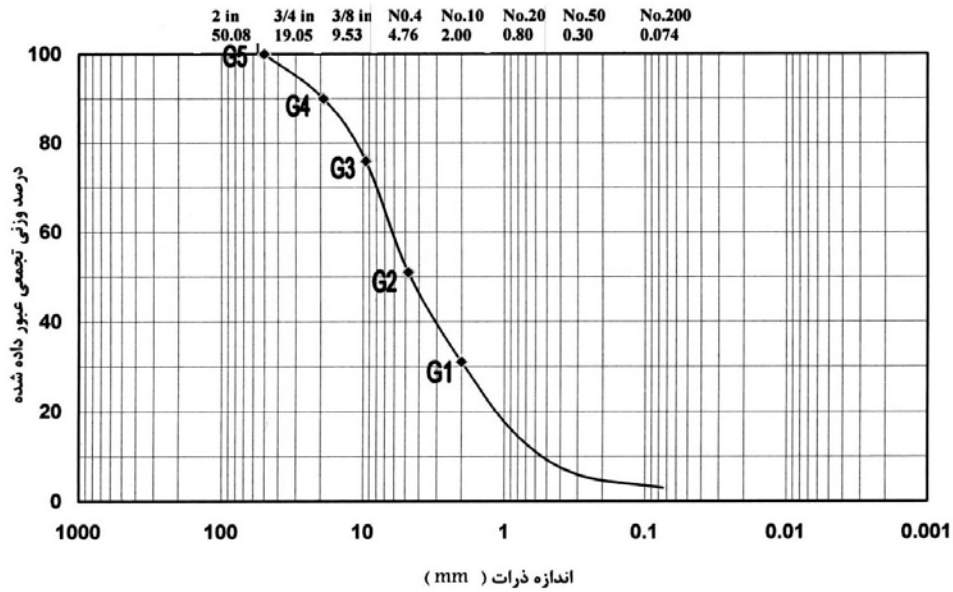
شکل ۸: منحنی دانه بندی مورد استفاده جهت تعیین نسبت تزریق پذیری [۱۴].
