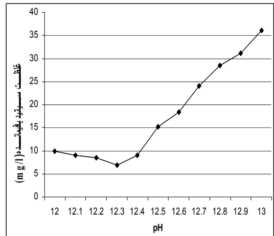
نمودار ۴: حذف سیانید با استفاده از محلول ۷۱ g/l هیپوکلریت کلسیم در pH=12-13 و دمای ۱۲ درجه سانتیگراد.
