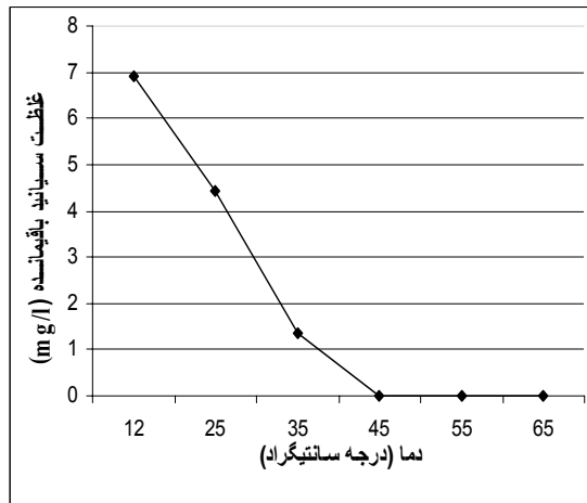
نمودار ۷: حذف سیانید با استفاده از محلول ۷۱٪ هیپوکلریت کلسیم در pH=12/3 و دمای (۱۲-۶۵) درجه سانتیگراد.
