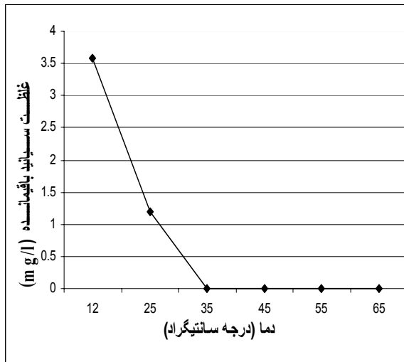
نمودار ۶: حذف سیانید با استفاده از محلول ۸۵٪ هیپوکلریت کلسیم در pH=12/3 و دمای (۱۲-۶۵) درجه سانتیگراد.
