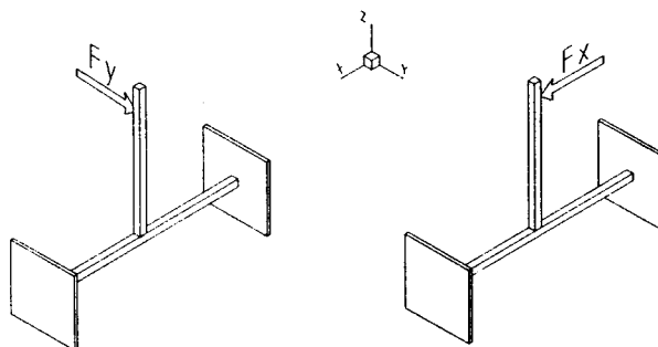
شکل ۱: جهات مهمترین بارهای وارده به اتصال مورد آزمایش.
