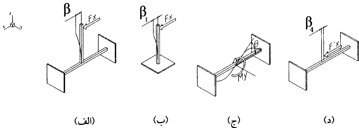
شکل ۳: فرآیند به دست آوردن مقدار سختی k_{\theta y} . (الف و ب): آزمایشهای شماره ۲ و ۴، (ج و د): گشتاور و نیروی ناشی از بار F_x در آزمایش شماره ۲.
