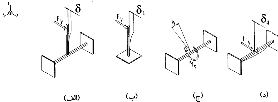
شکل ۲: فرآیند به دست آوردن مقدار سختی k_{\theta x} . (الف و ب): آزمایشهای شماره ۱ و ۲، (ج و د): گشتاور و نیروی ناشی از بار F_y در آزمایش شماره ۱.
