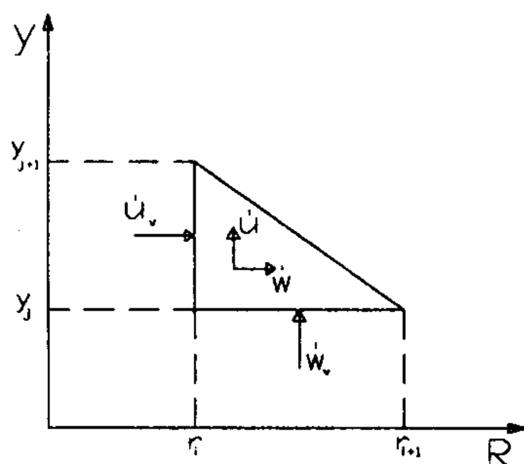
شکل ۷: المان رینگی مثلثی (محور متقارن).
