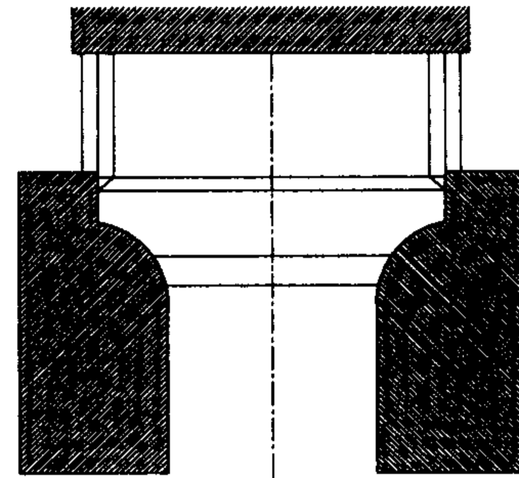
شکل ۱۴: پیشروی فرآیند اکستروژن فورجینگ.
