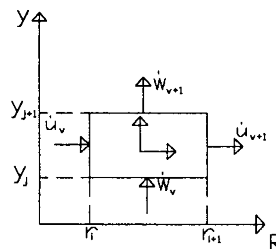
شکل ۶: المان رینگی چهارگوش (محور متقارن).
