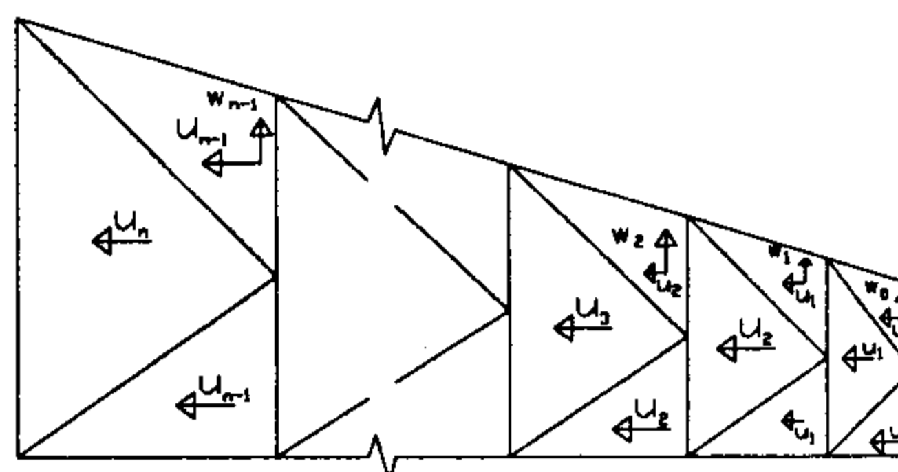
شکل ۵: نمونه ای از المان ذوزنقه ای و تقسیم آن به سلول ها و مثلث های صلب (کرنش مسطح).
