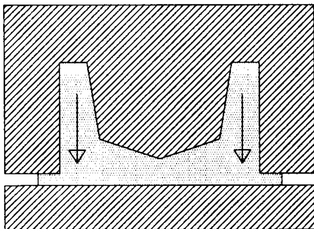
شکل ۱۷: مرحله نهائی فرآیند آهنگری محور متقارن (پر شدن کامل حفره های قالب).
