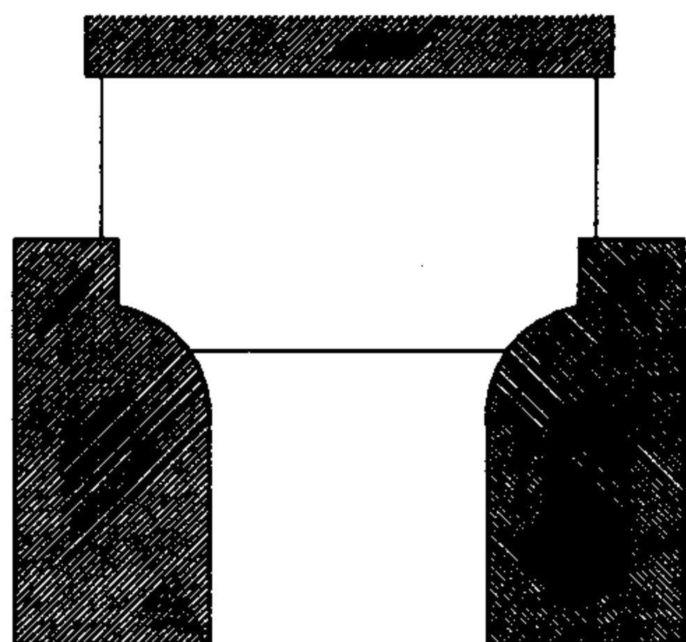
شکل ۱۱: آهنگری کرنش مسطح - فرآیند فورجینگ اکستروژن.
