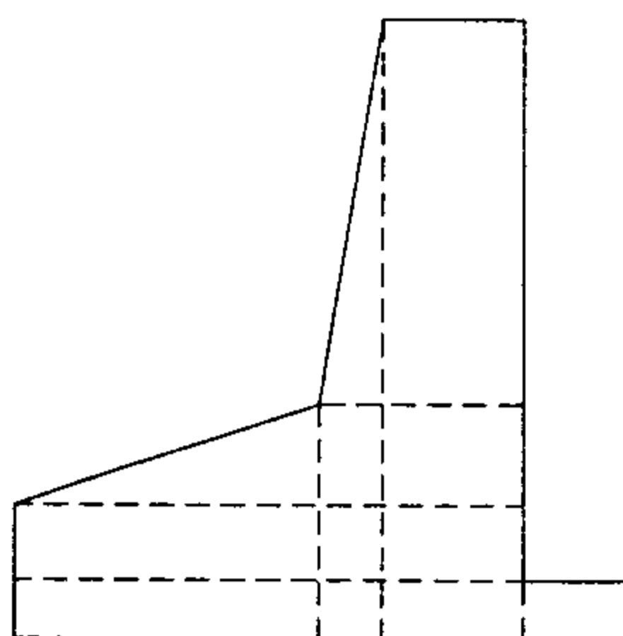
شکل ۱۸: المان بندی سطح مقطع با ۱۲ المان (فرایند آهنگری محور متقارن).
