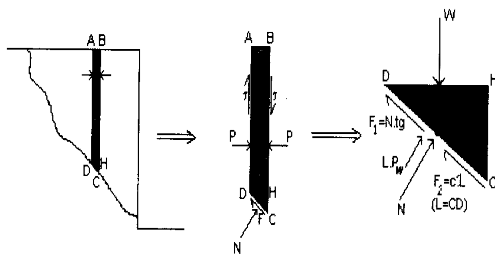
شکل ۲: آنالیز نیروها در یک المان از خاک.
