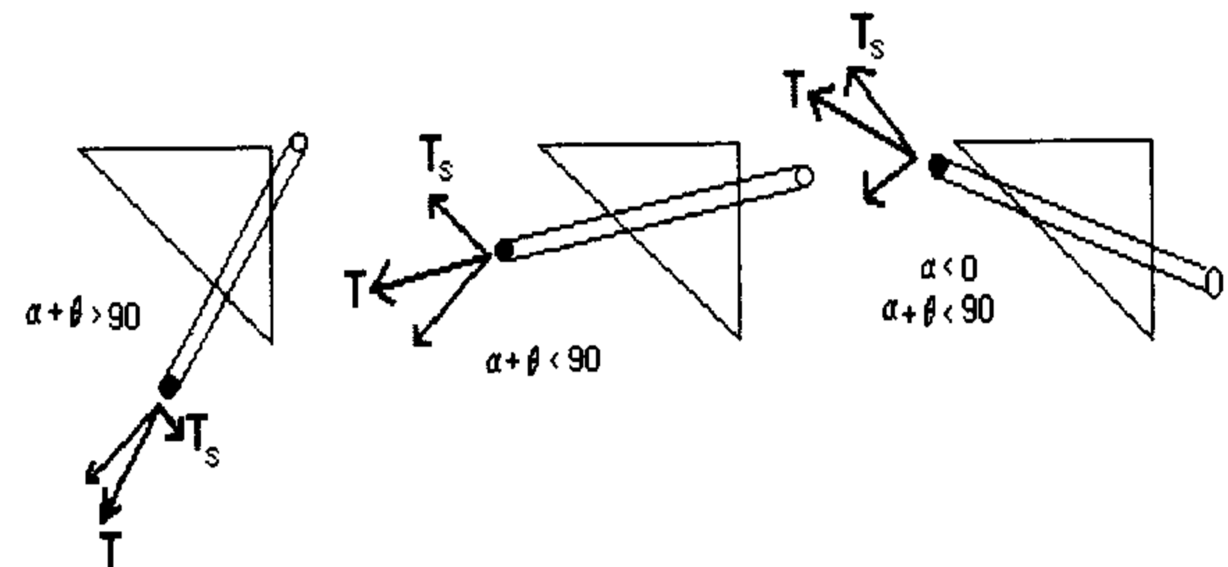
میخ با کارایی زیاد میخ با کارایی کم میخ با کارایی منفی
