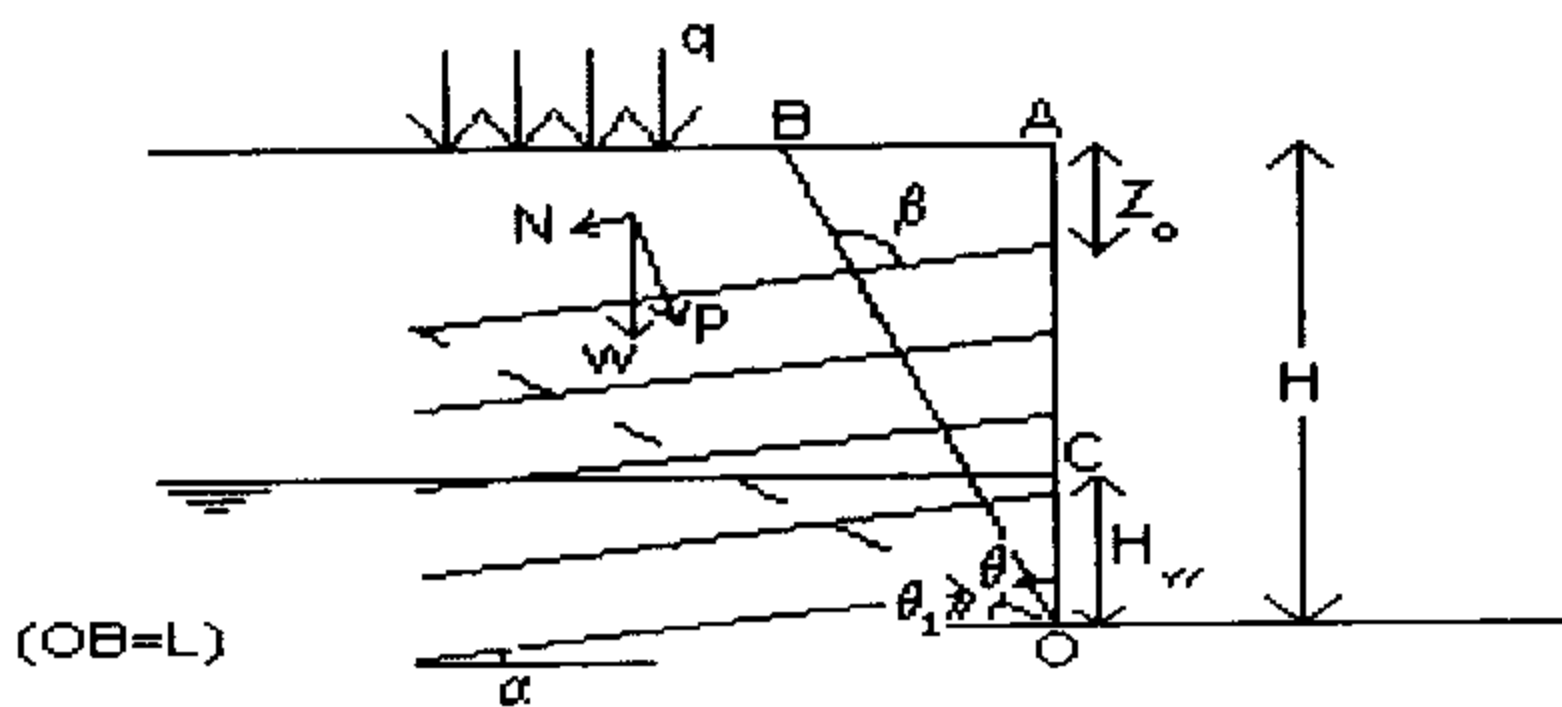
شکل ۱: سطح گسیختگی و جزئیات در روش Luo و همکاران.
