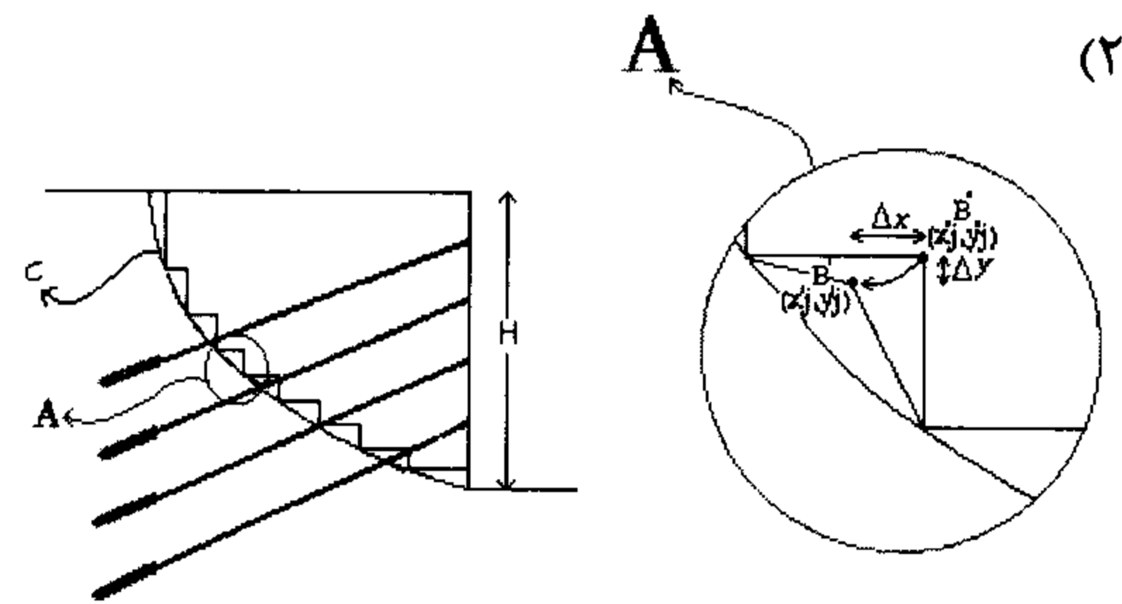
شکل ۶: نحوه حرکت یک گره اختیاری مانند B
