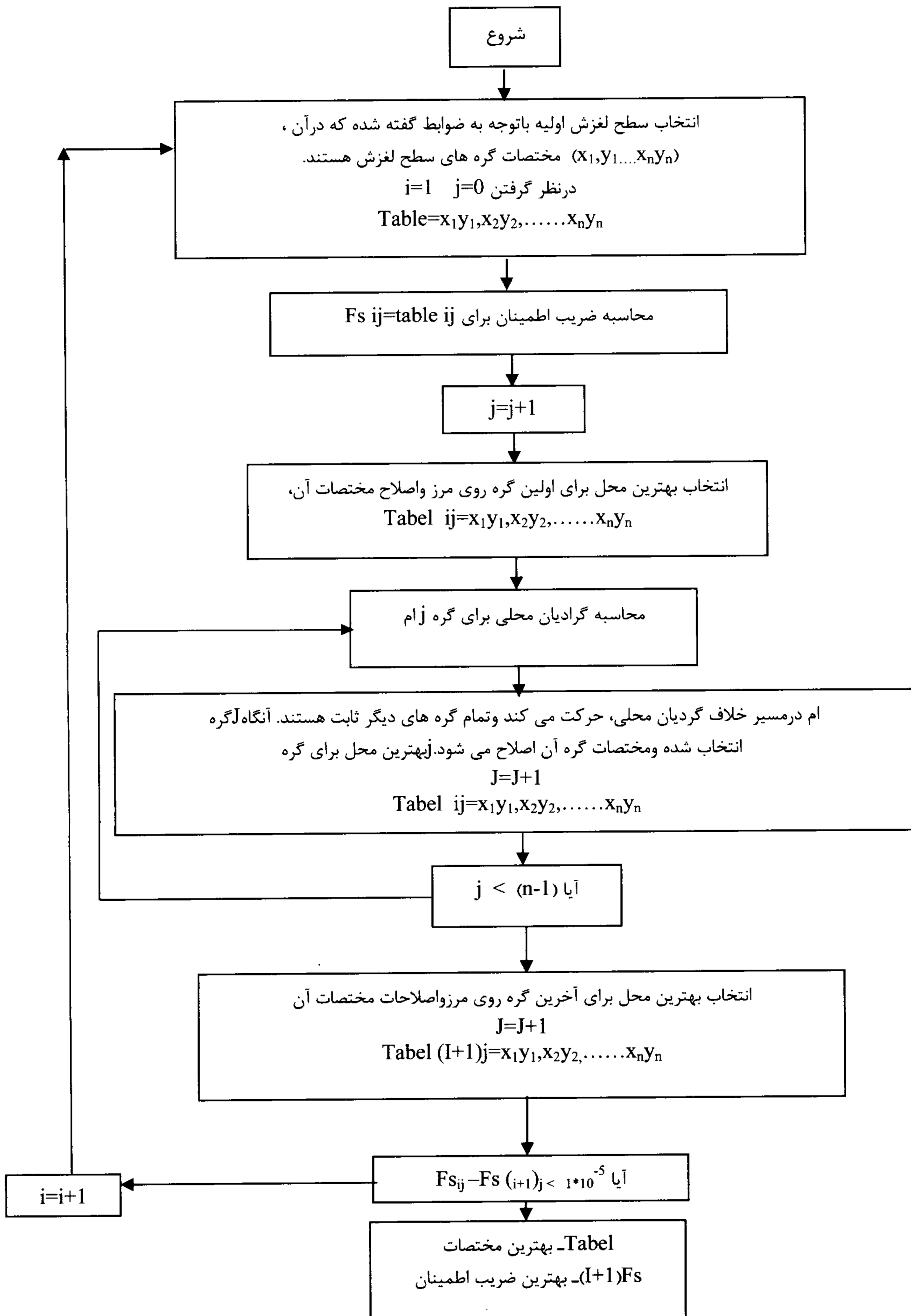
شکل ۷: فلوجارت برنامه رایانه ای.
