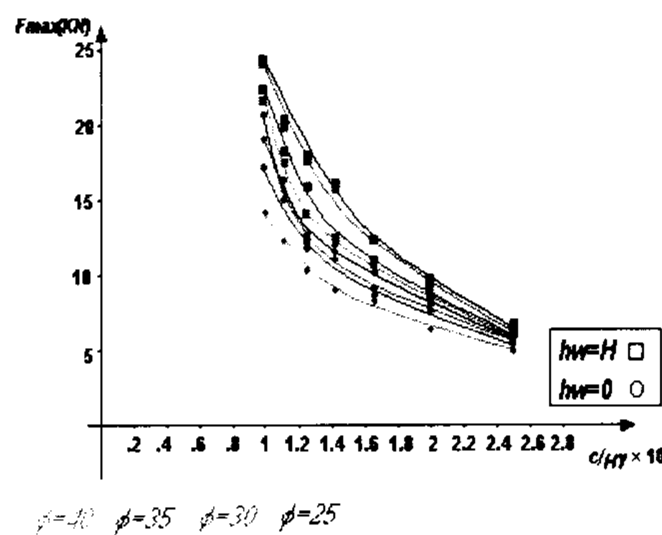
شکل ۱۰: تاثیر \phi و C/\gamma H روی حداکثر نیروی کششی ایجاد شده در میخ.
