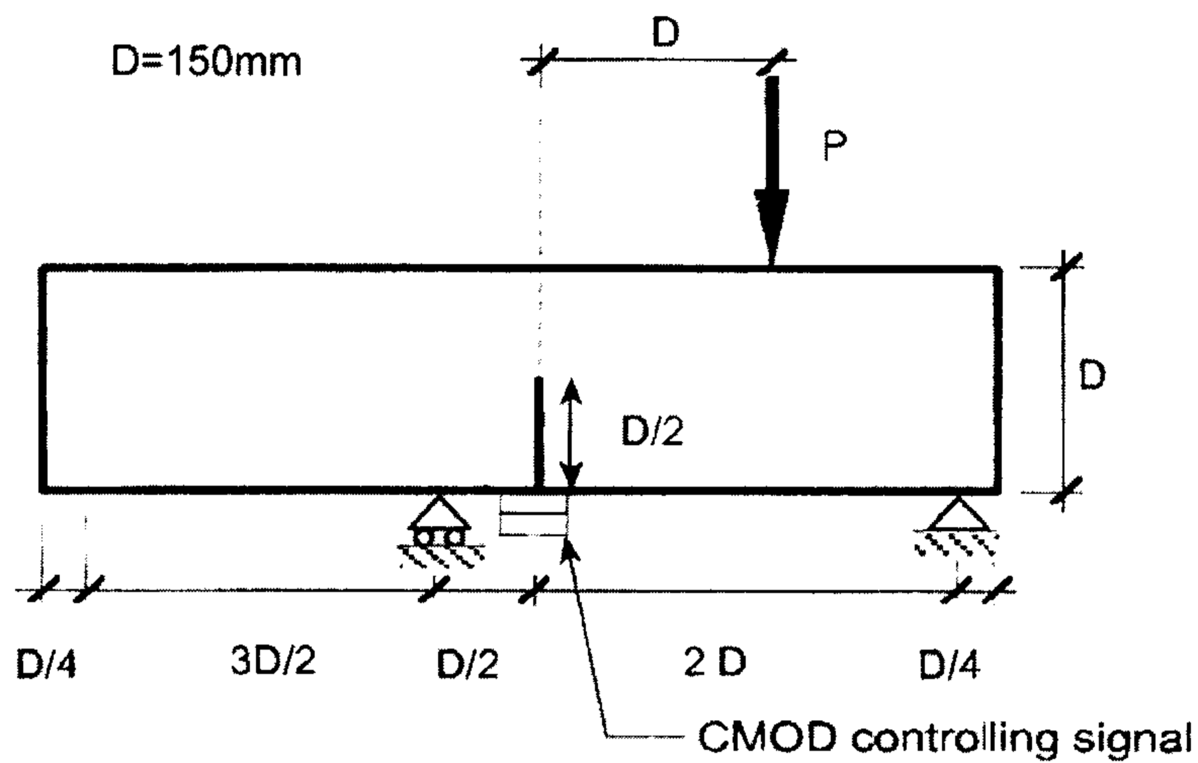
شکل ۶: ابعاد مدل شماره یک [۱۰].
