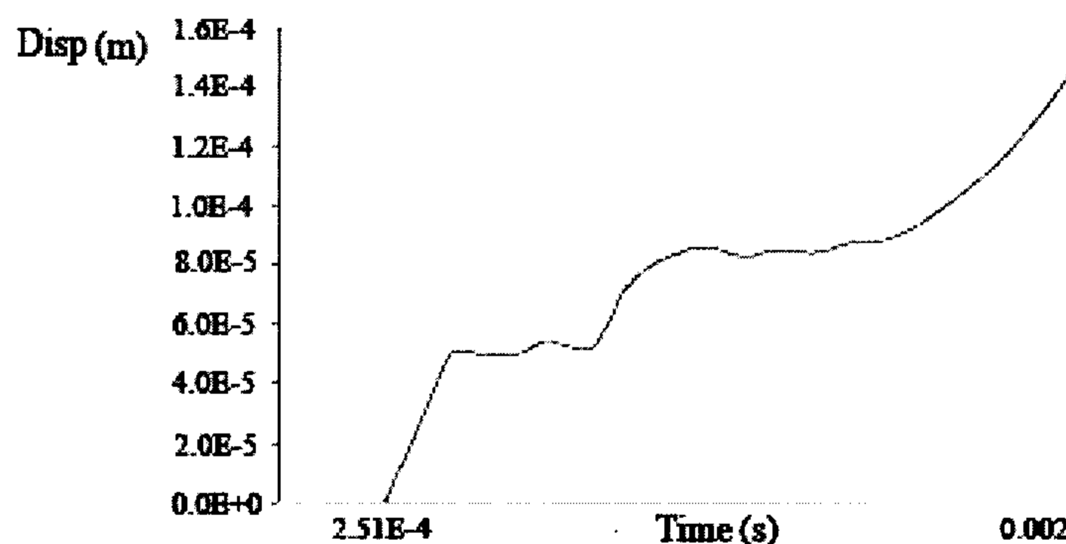
شکل ۲۲: نمودار تغییر مکان قائم وسط دهانه.
