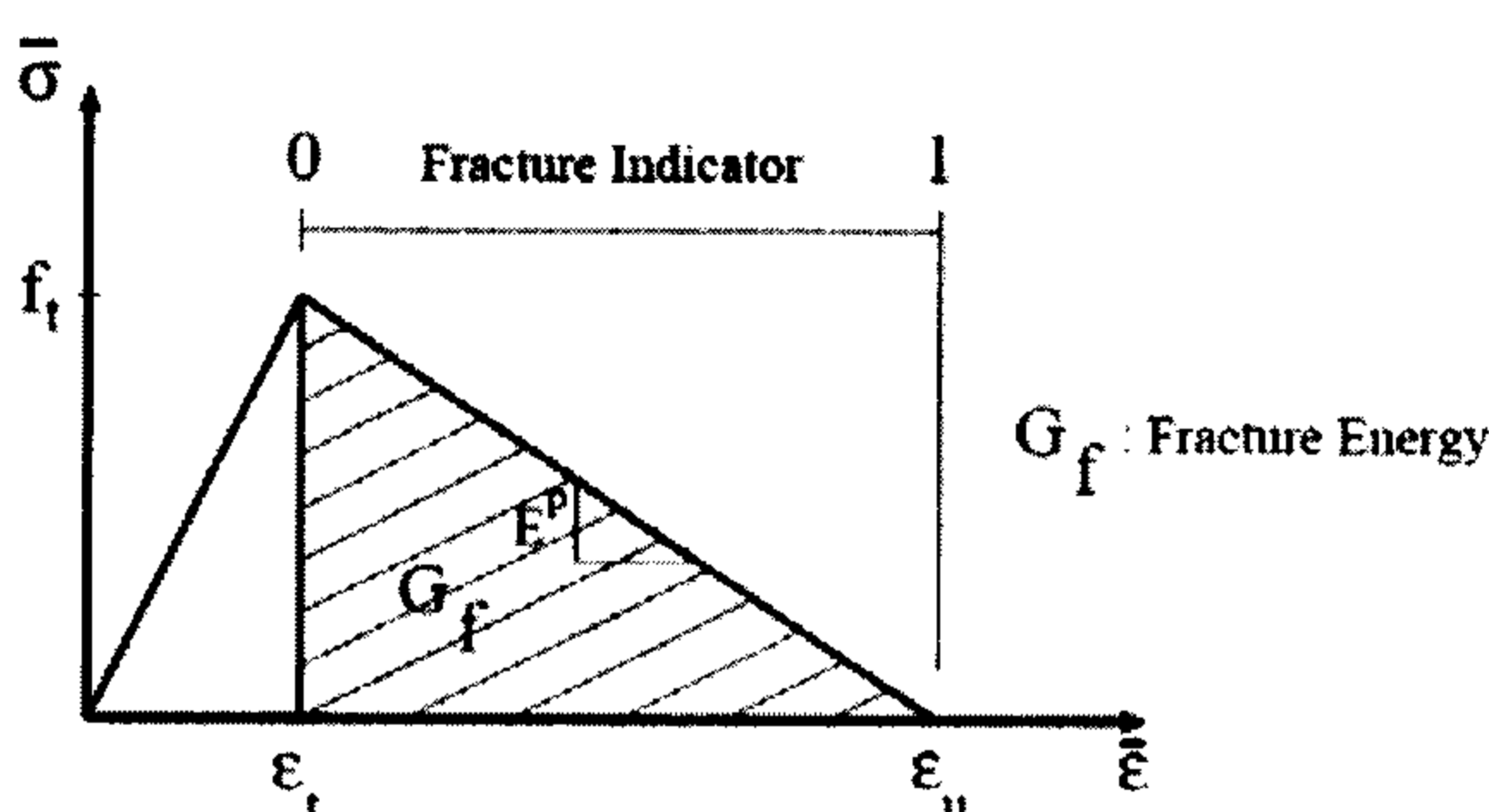
شکل ۲: مدل نرم شدگی انرژی شکست [۱۸].
