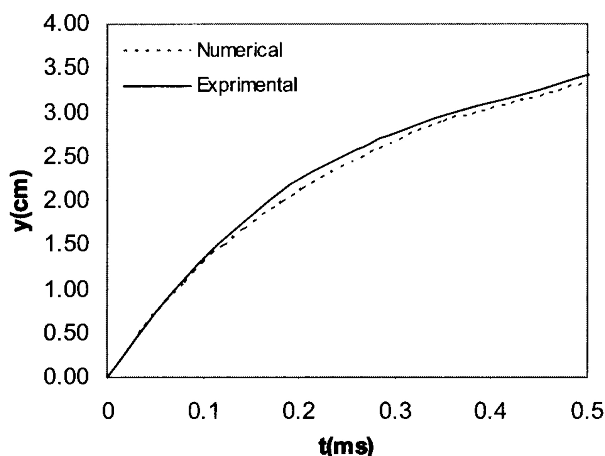
شکل ۱۵: منحنی نفوذ پرتابه بر حسب زمان.
