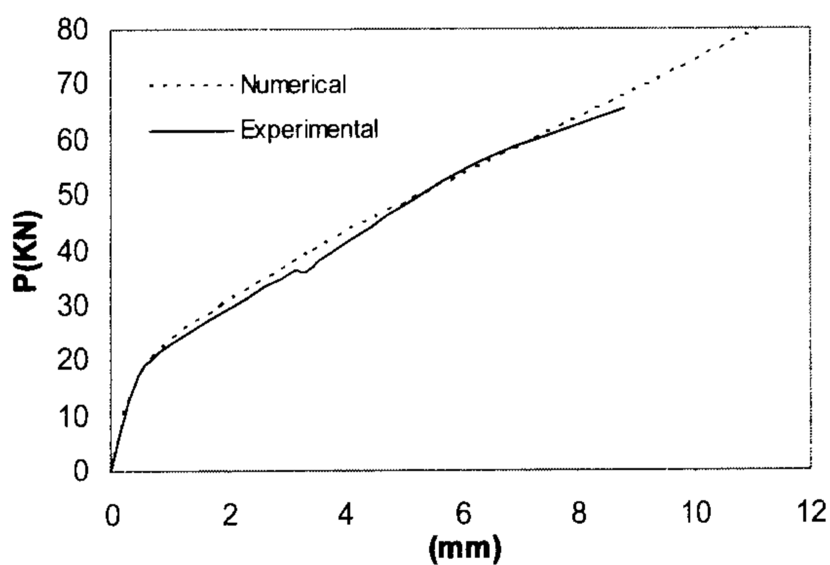
شکل ۱۱: منحنی تغییر مکان وسط دهانه تیر.
