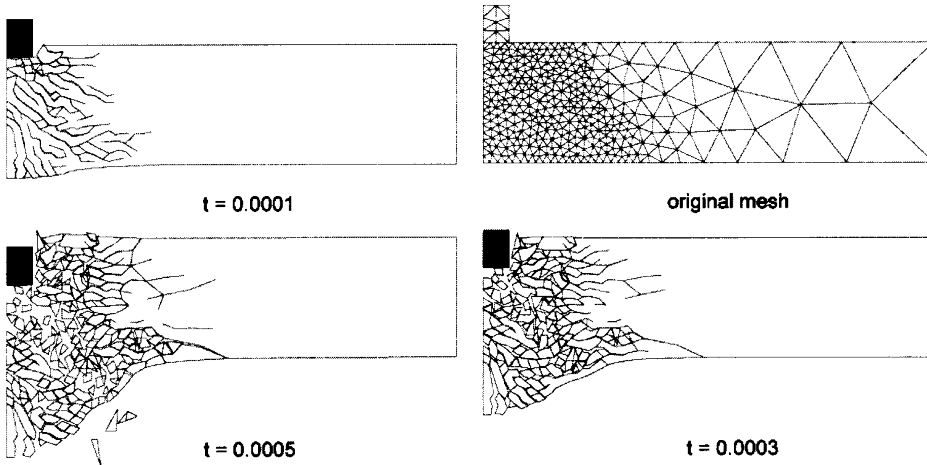
شکل ۱۷: الگوی گسترش ترک پس از برخورد پرتابه.
