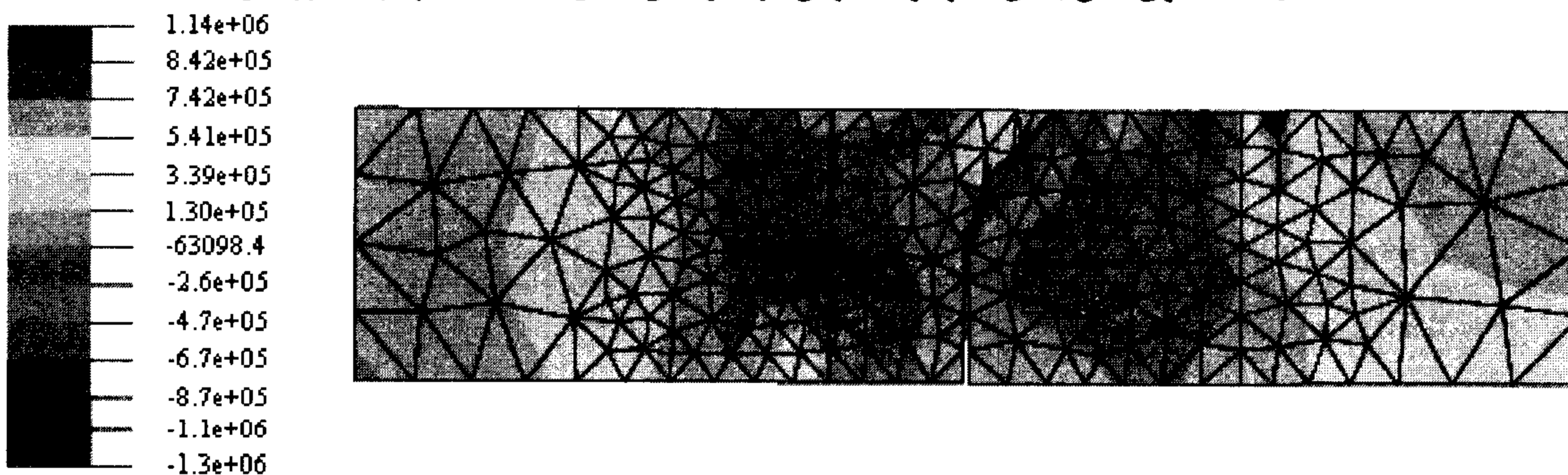
شکل ۸: توزیع تنش برشی \tau_{xy} .
