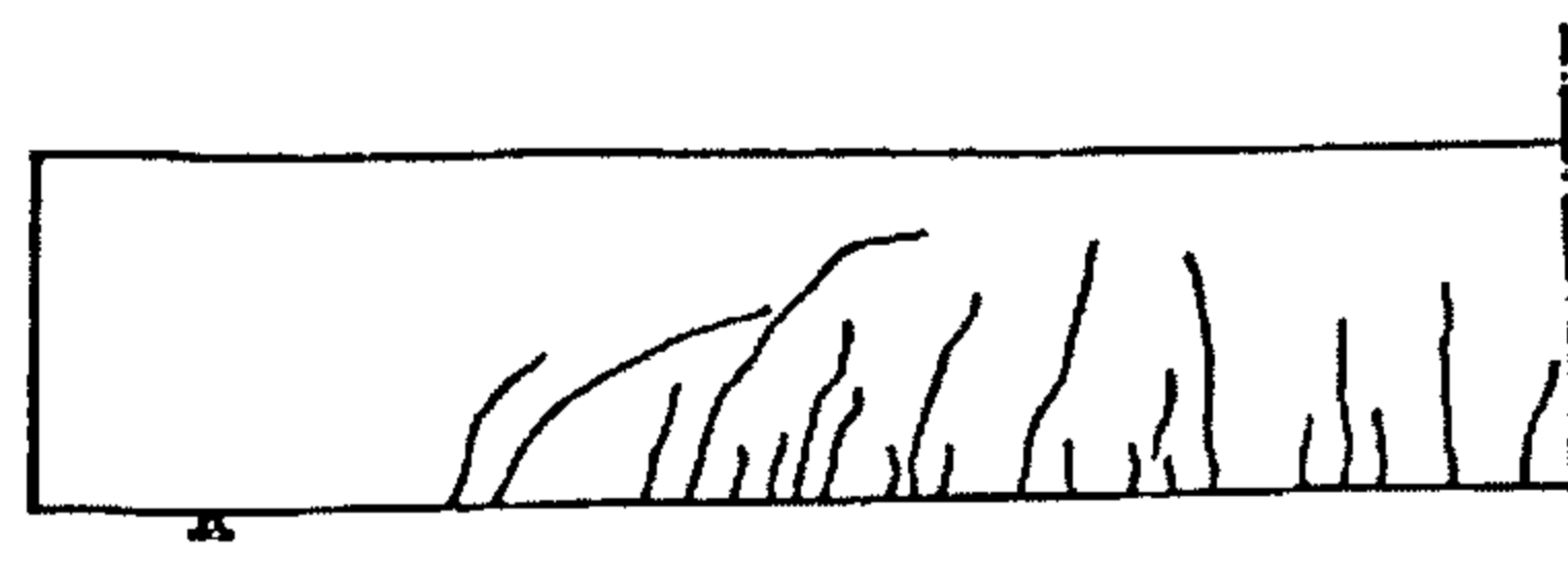
شکل ۱۲: شکل ترک خوردگی آزمایشگاهی [۸].
