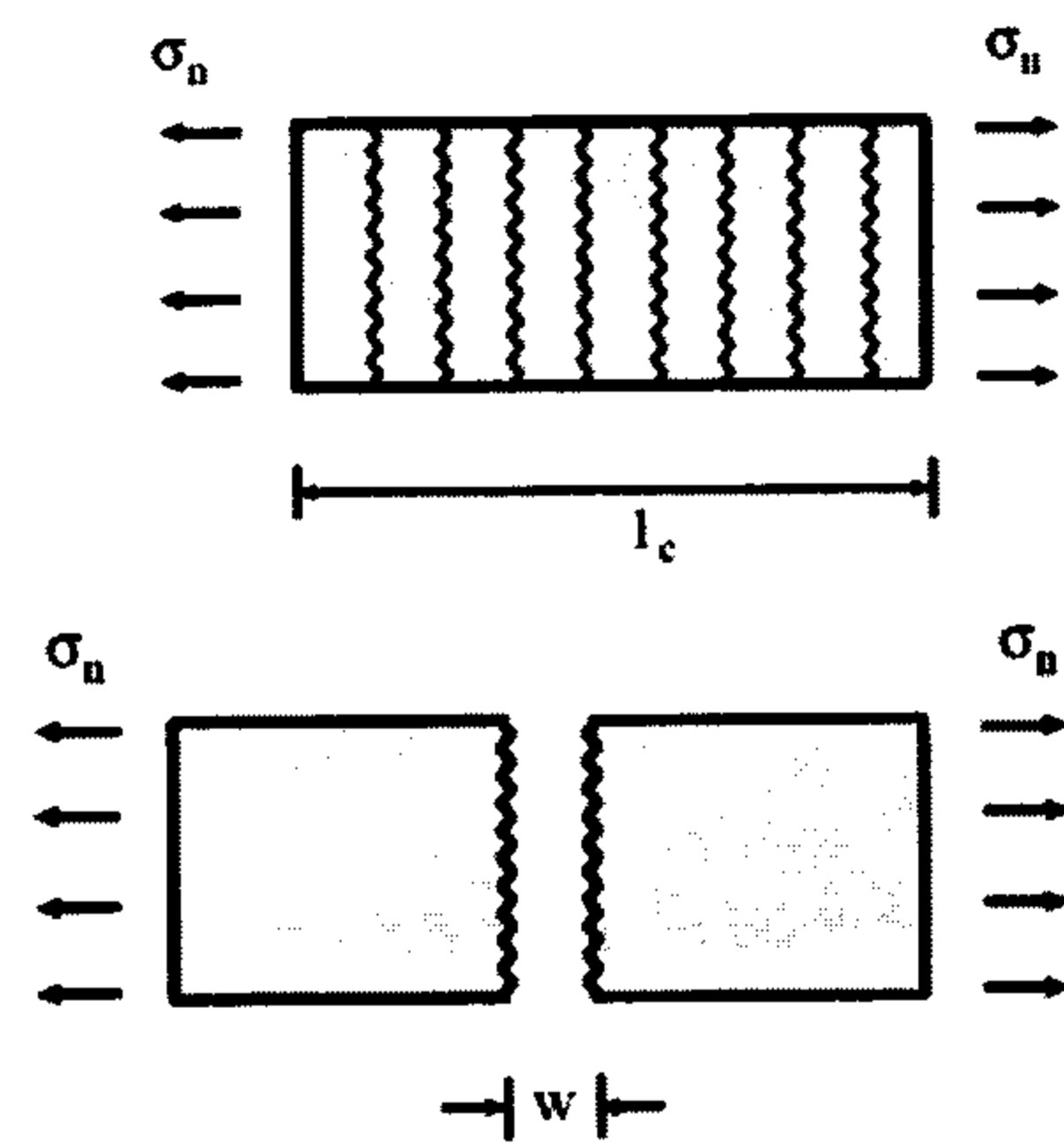
شکل ۳: مدل‌های ترک پیوسته و مجزا.
