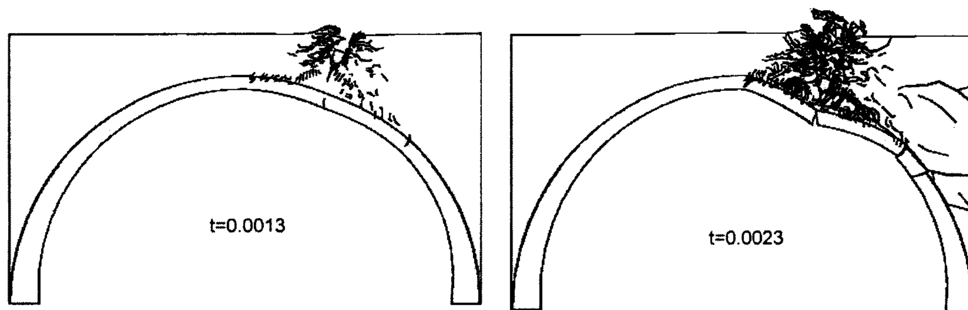
شکل ۲۴: الگوی گسترش ترک در زمانهای t=0.0013 \text{ s} و t=0.0023 \text{ s} .
