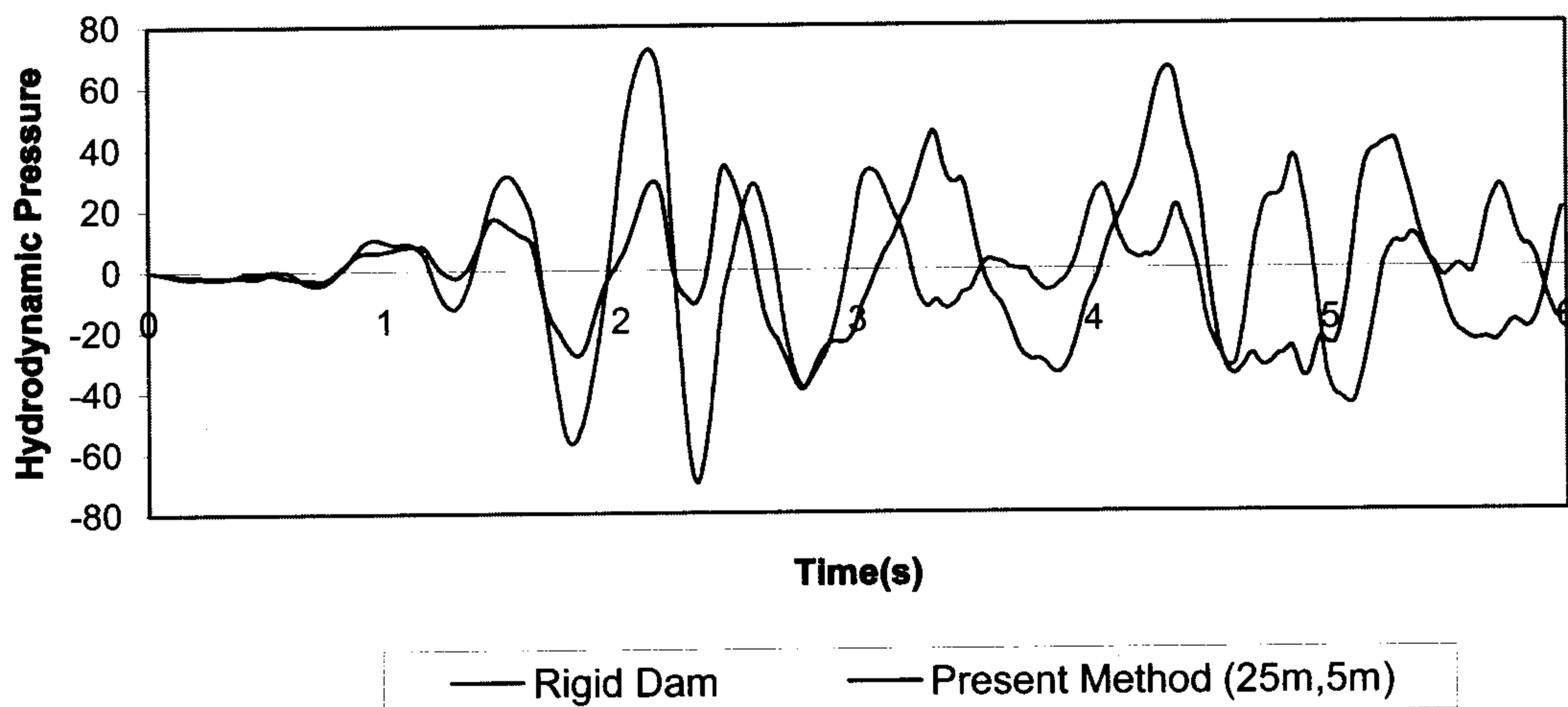
شکل ۱۳: تاثیر صلب در نظر گرفتن سد در فشار هیدرودینامیک.
