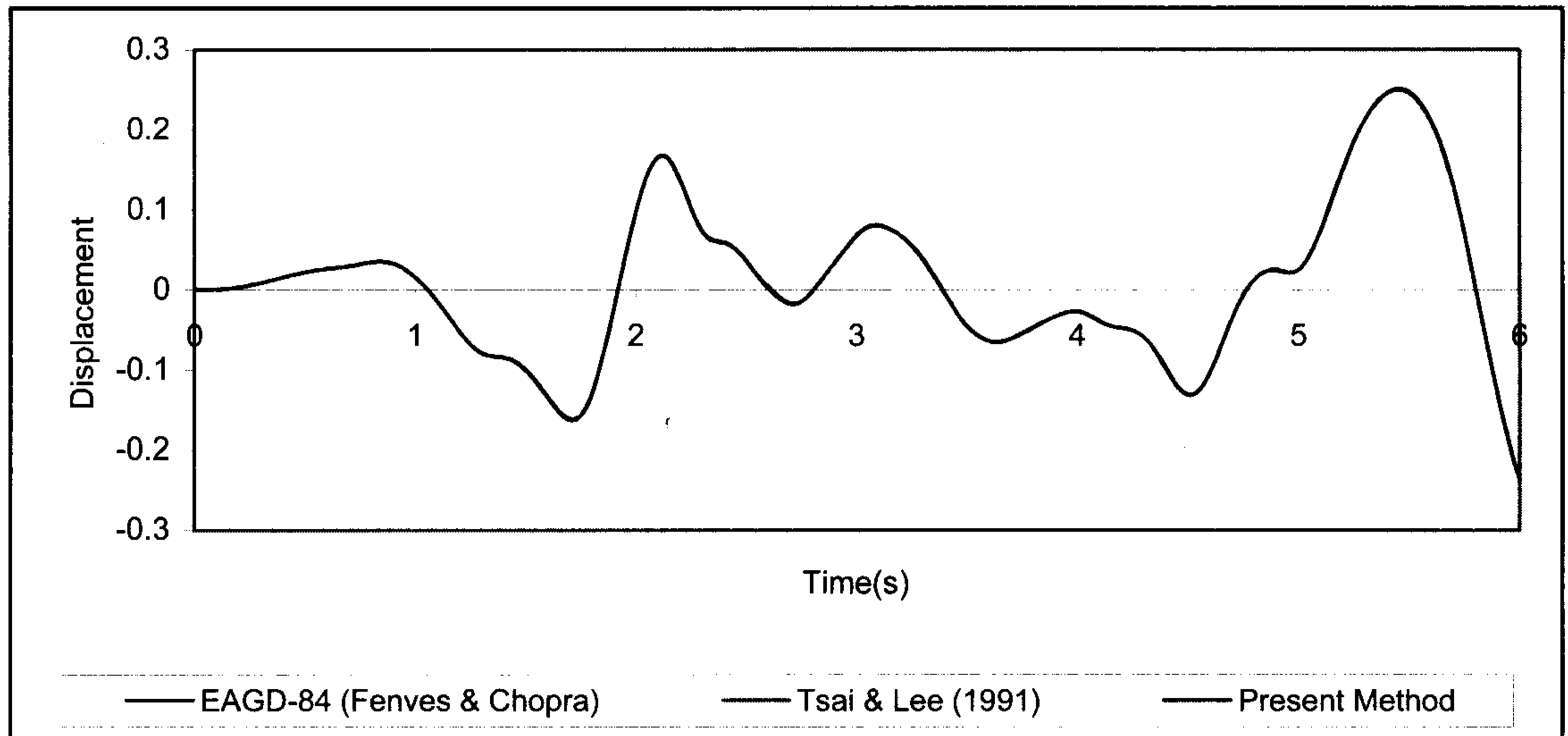
شکل ۲: تغییر مکان تاج سد در حالت پر در زلزله ال-سنترال از روش پیشنهادی، روش Tsai & Lee و برنامه EAGD-84.
