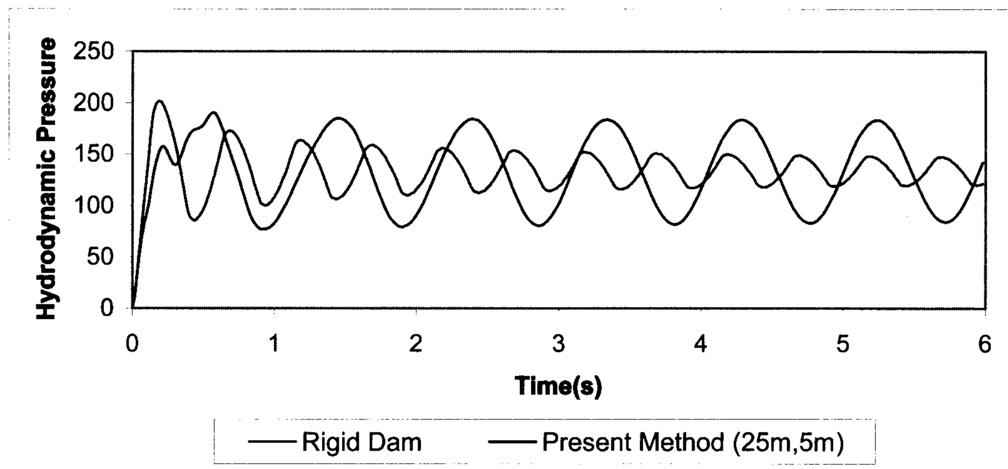
شکل ۱۴: تاثیر صلب در نظر گرفتن سد در فشار هیدرودینامیک.
