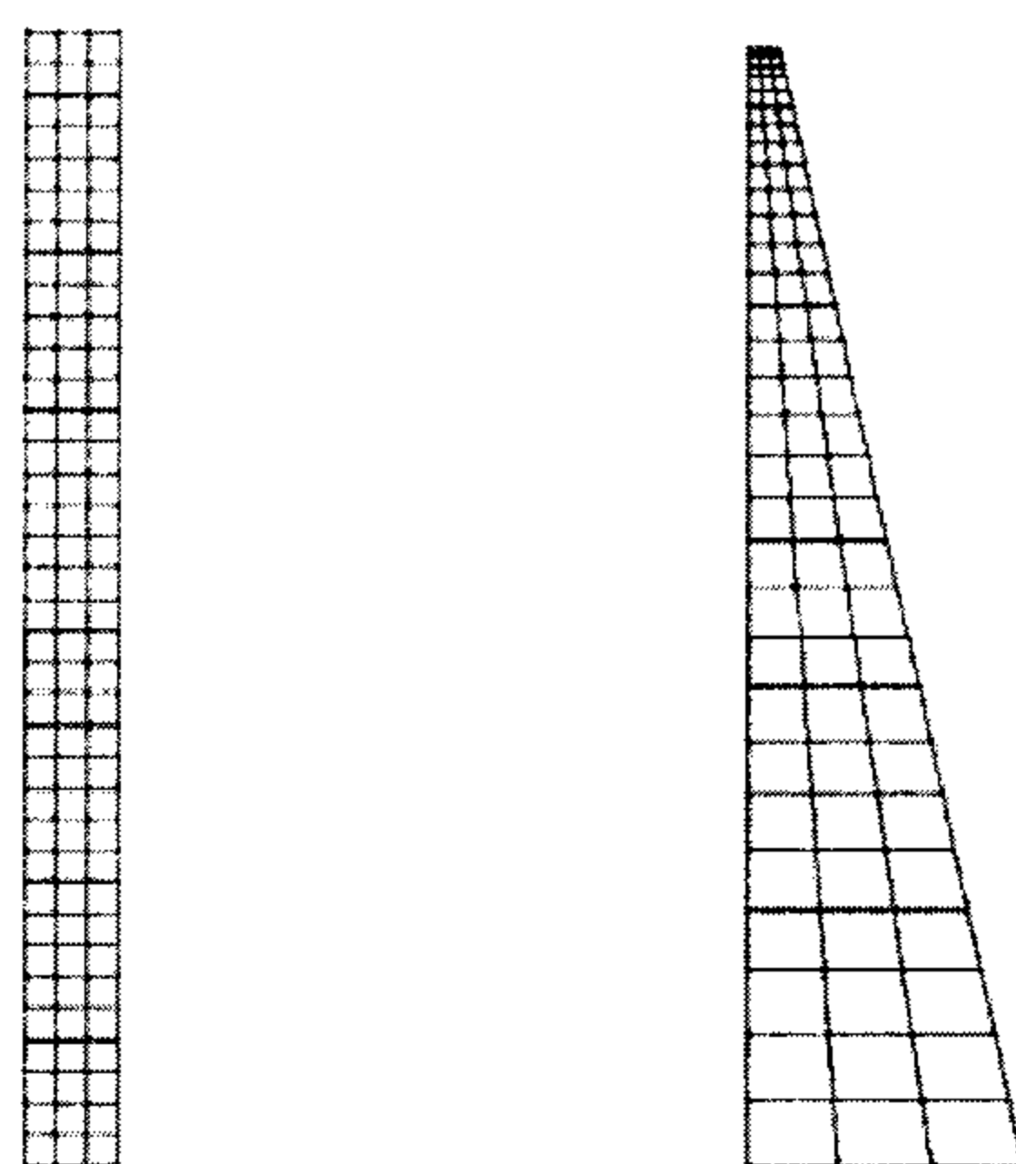
شکل ۱۵: شبکه المانهای برنامه EAGD-84 مثالهای ۲ و ۳.
