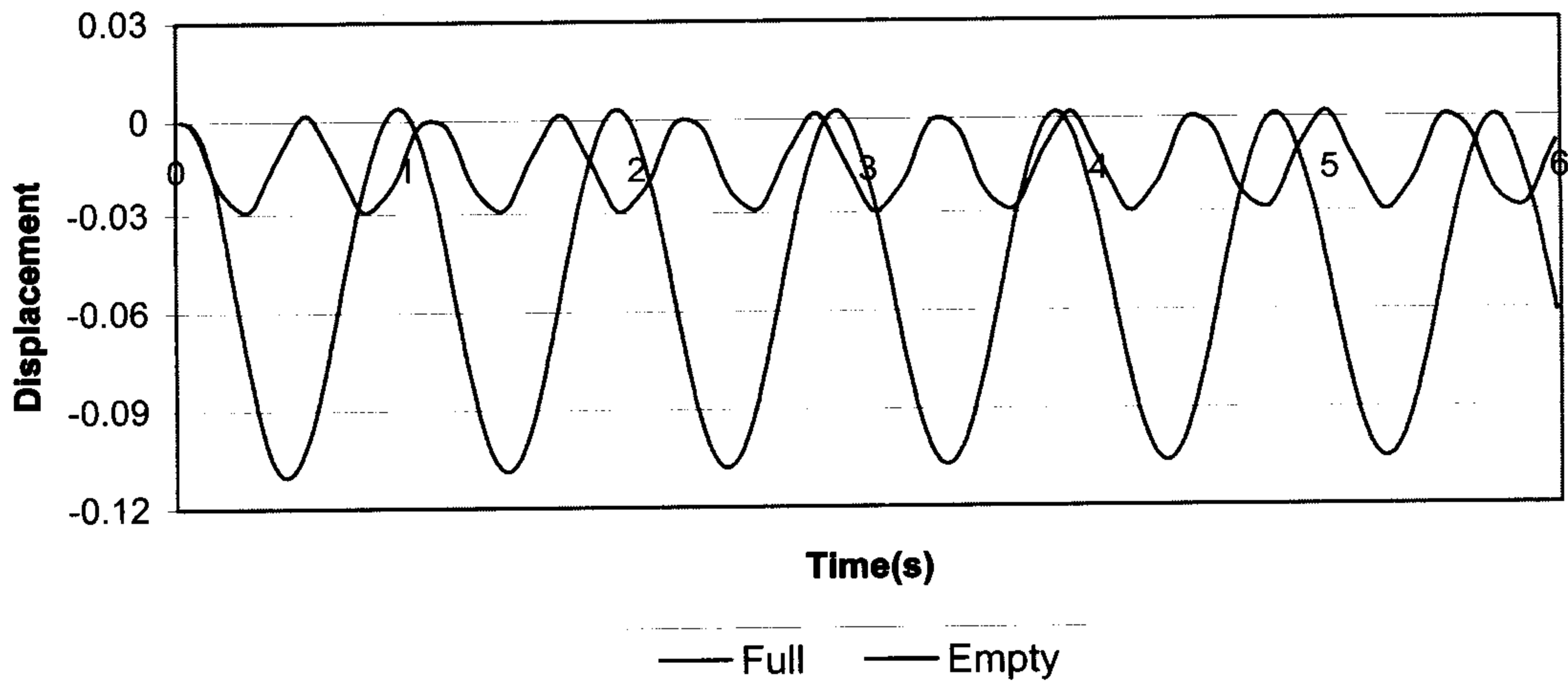
شکل ۱۲: مقایسه تغییر مکان تاج سد با ضخامت متغیر حالت پر و خالی تحت شتاب ثابت 1 m/s^2 بر حسب زمان.
