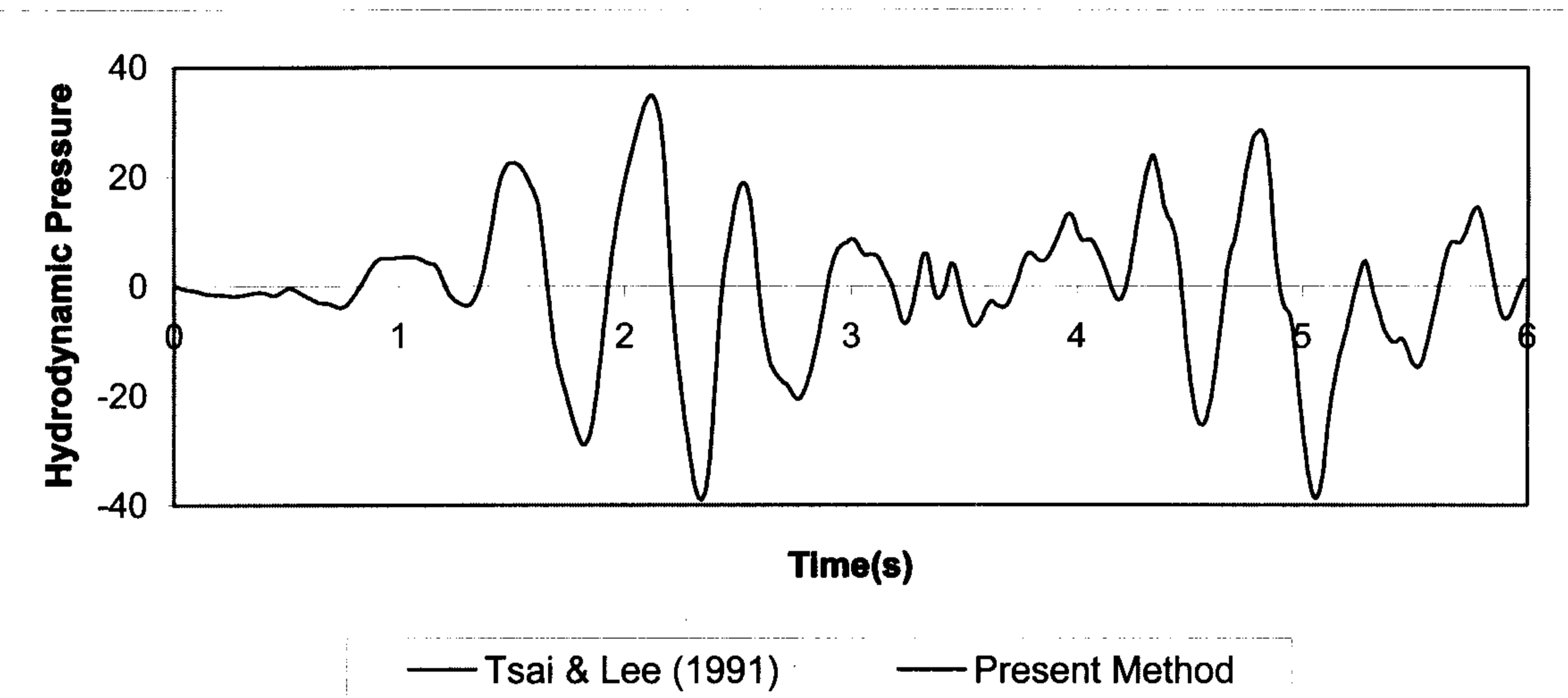
شکل ۴: فشار هیدرودینامیک در پایین ترین نقطه سد تحت زلزله ال سنترال برحسب زمان.
