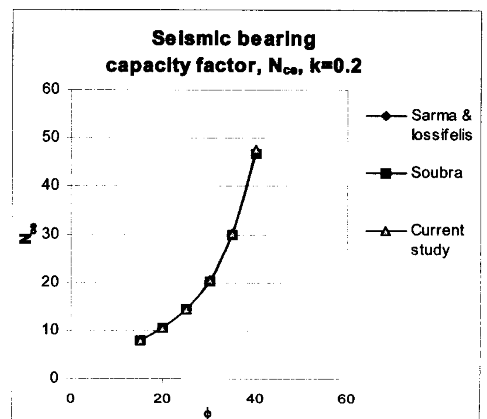
شکل ۵: مقایسه ضریب ظرفیت باربری N_{ce} برای K=0.2
