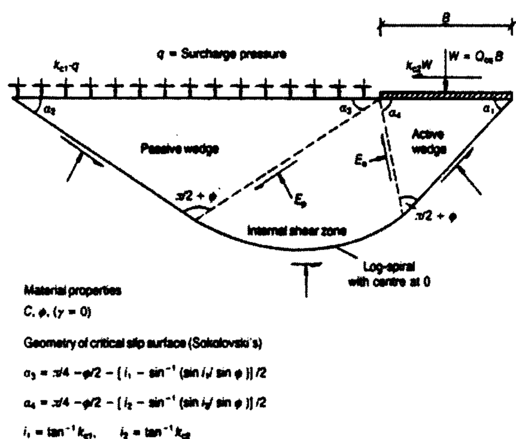
شکل ۲: جزئیات مکانیزم مورد استفاده توسط سارما و یوسفیلِس (Sarma & Iossifelis 1998).
