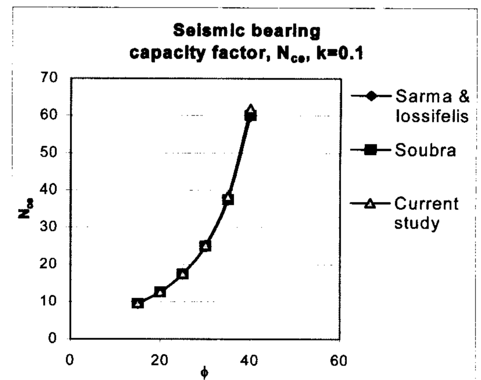
شکل ۴: مقایسه ضریب ظرفیت باربری N_{ce} برای K=0.1
