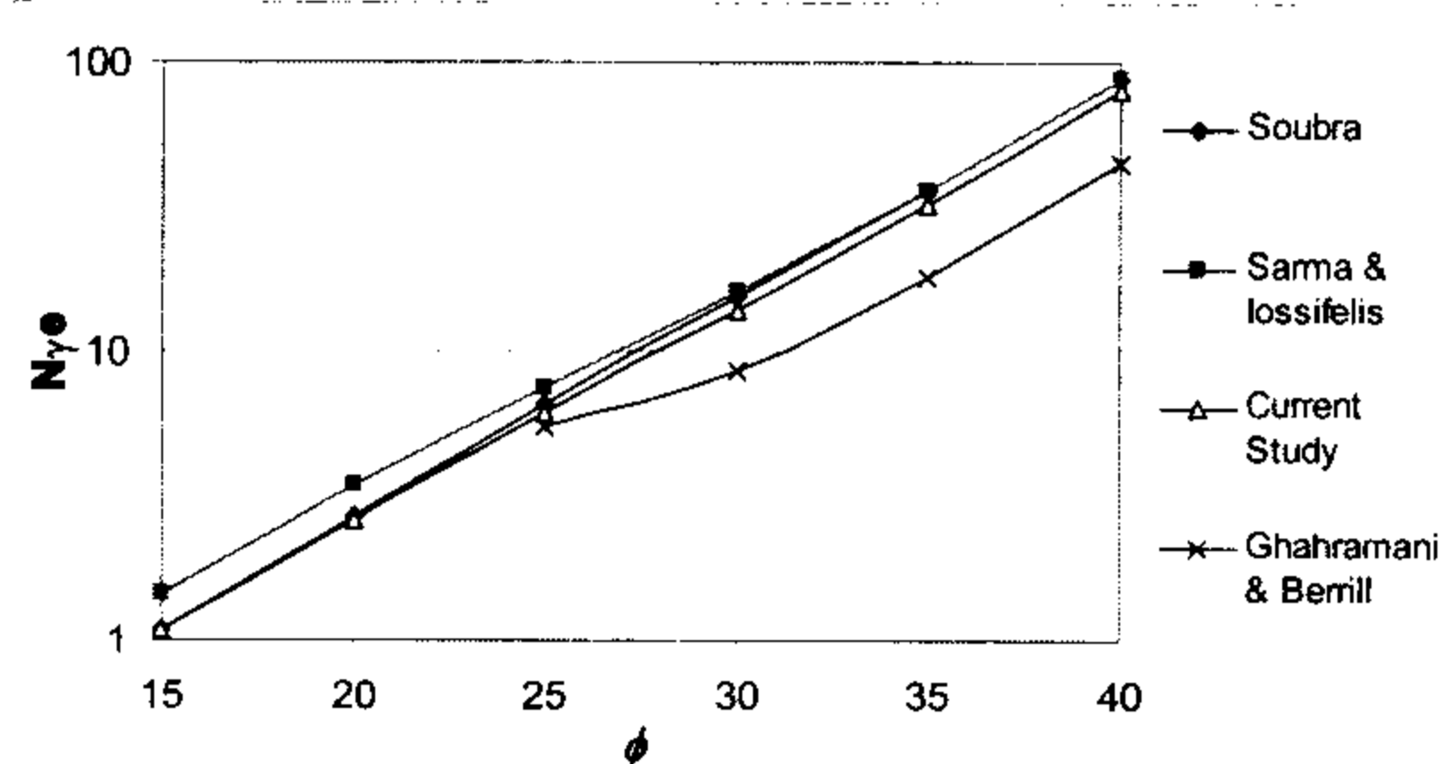
شکل ۷: نمودار ضریب ظرفیت باربری لرزه‌ای N_{ye} برای K = 0.1
