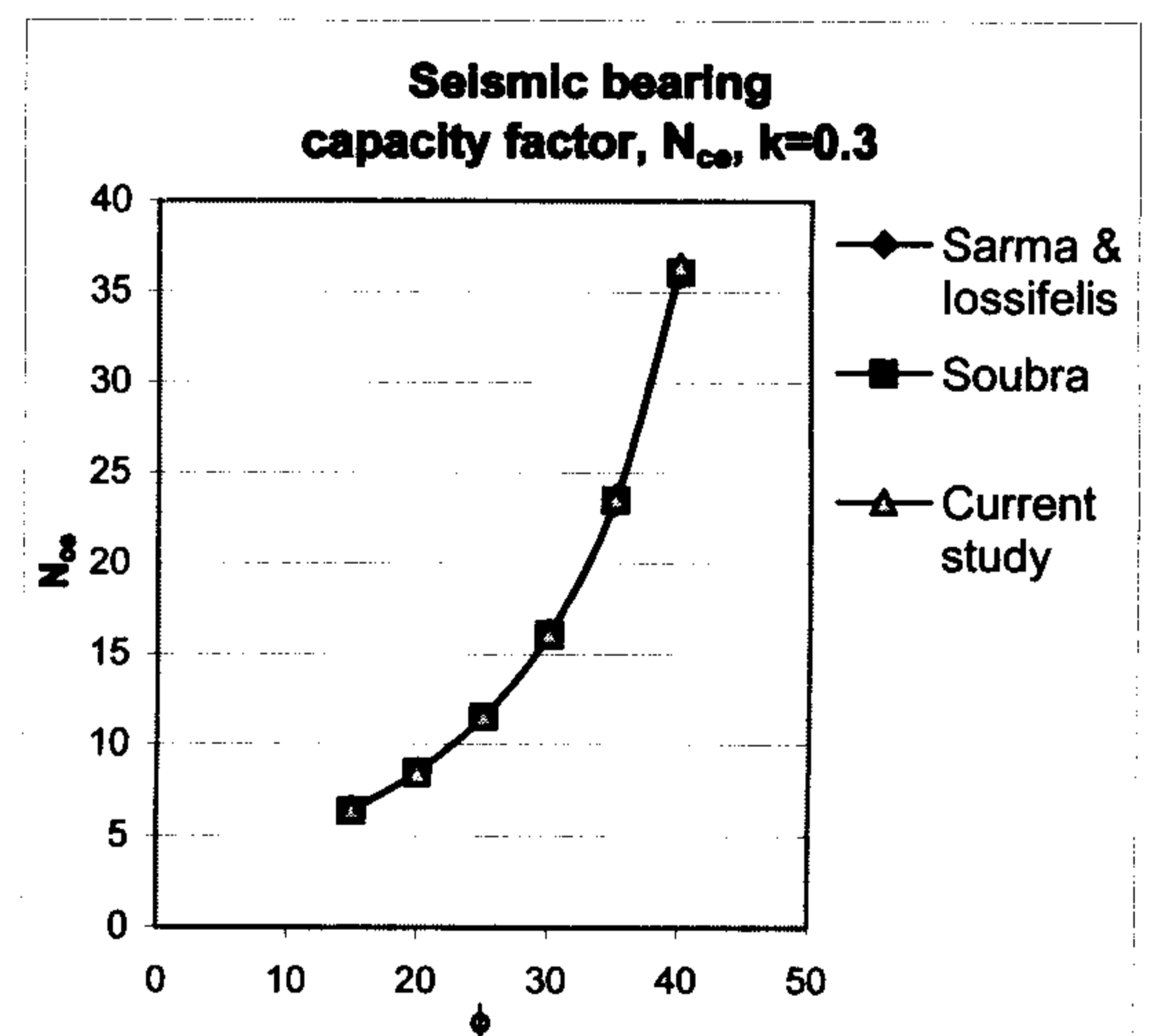
شکل ۶: مقایسه ضریب ظرفیت باربری N_{ce} برای K=0.3
