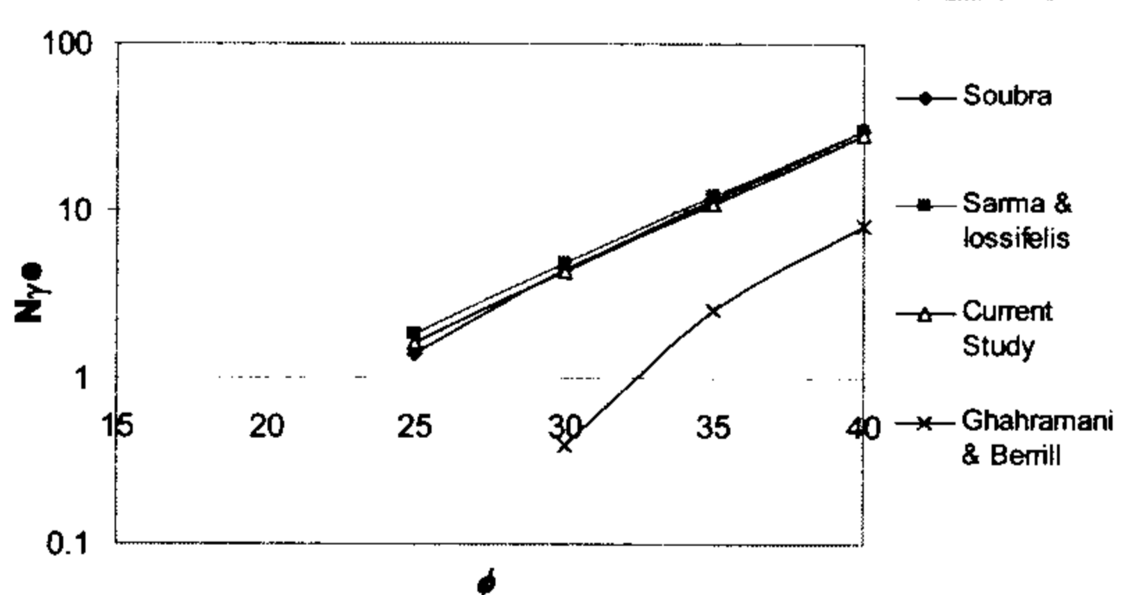
شکل ۹: نمودار ضریب ظرفیت باربری لرزه‌ای N_{ye} برای K = 0.3
