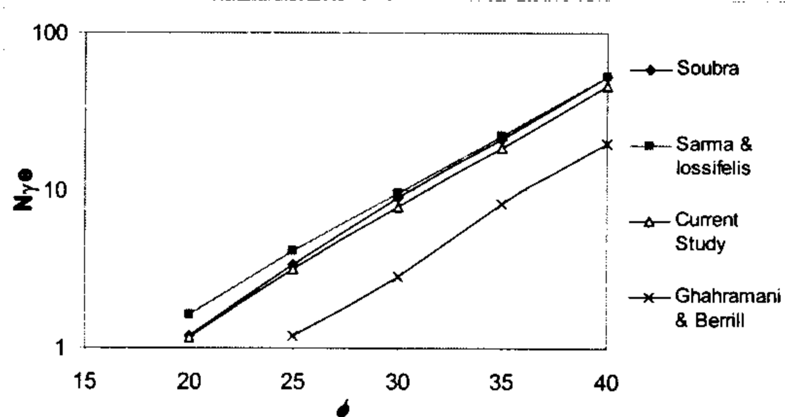
شکل ۸: نمودار ضریب ظرفیت باربری لرزه‌ای N_{ye} برای K = 0.2
