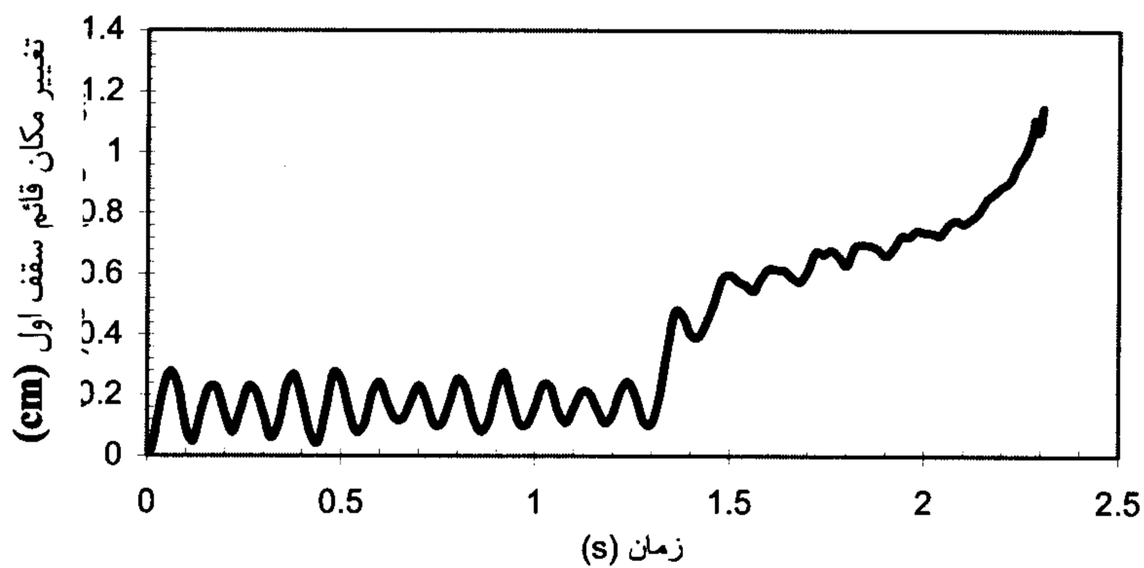
شکل ۸: تغییر مکان قائم سقف اول در اثر مولفه افقی شتاب نداشت زلزله ناغان.
