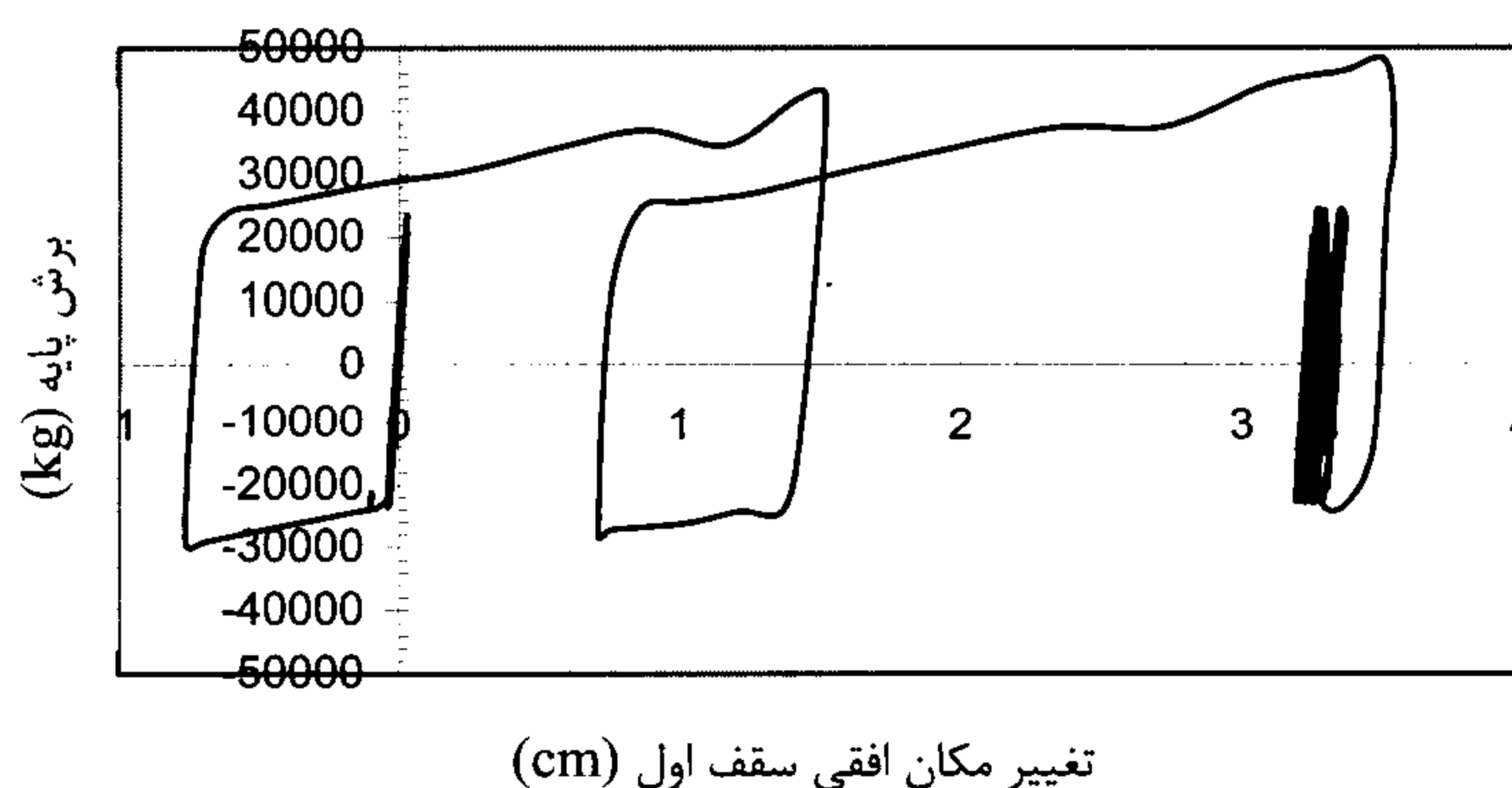
شکل ۱۸: منحنی برش پایه - تغییر مکان طبقه اول قاب خرجینی مقاوم شده تحت زلزله نورتریج.
