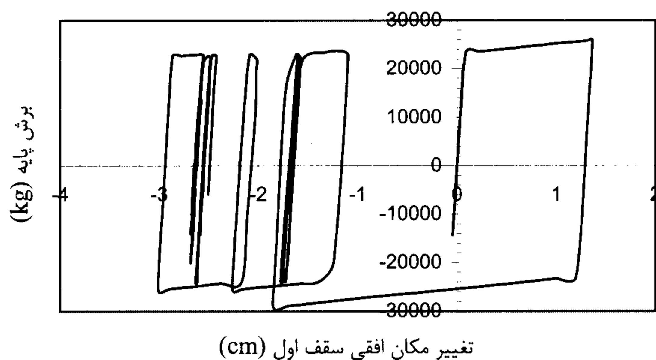
شکل ۱۷: منحنی برش پایه - تغییر مکان طبقه اول قاب خرجینی مقاوم شده تحت زلزله ناغان.
