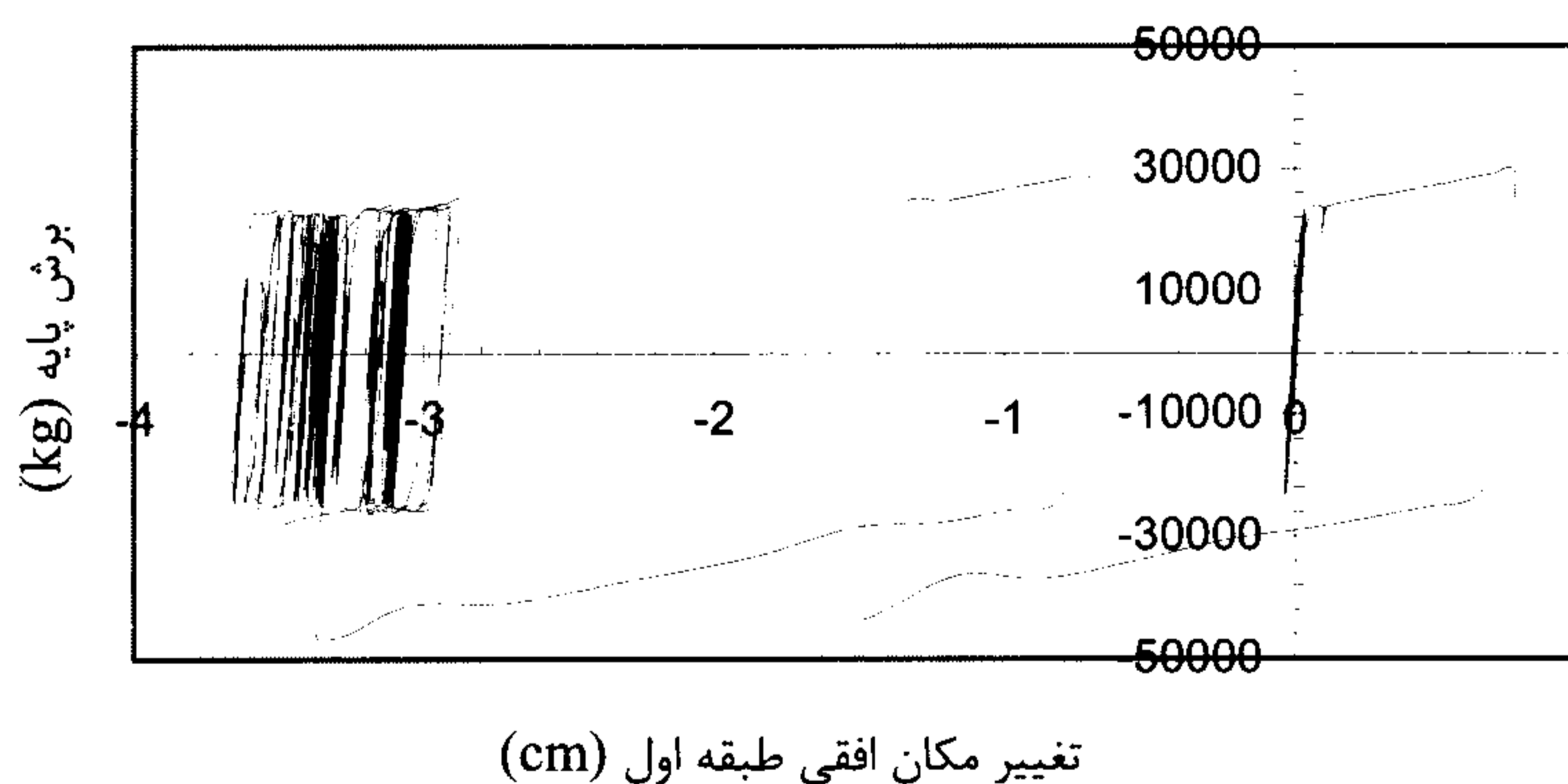
شکل ۱۹: منحنی برش پایه - تغییر مکان طبقه اول قاب خرجینی مقاوم شده تحت زلزله طبس.
