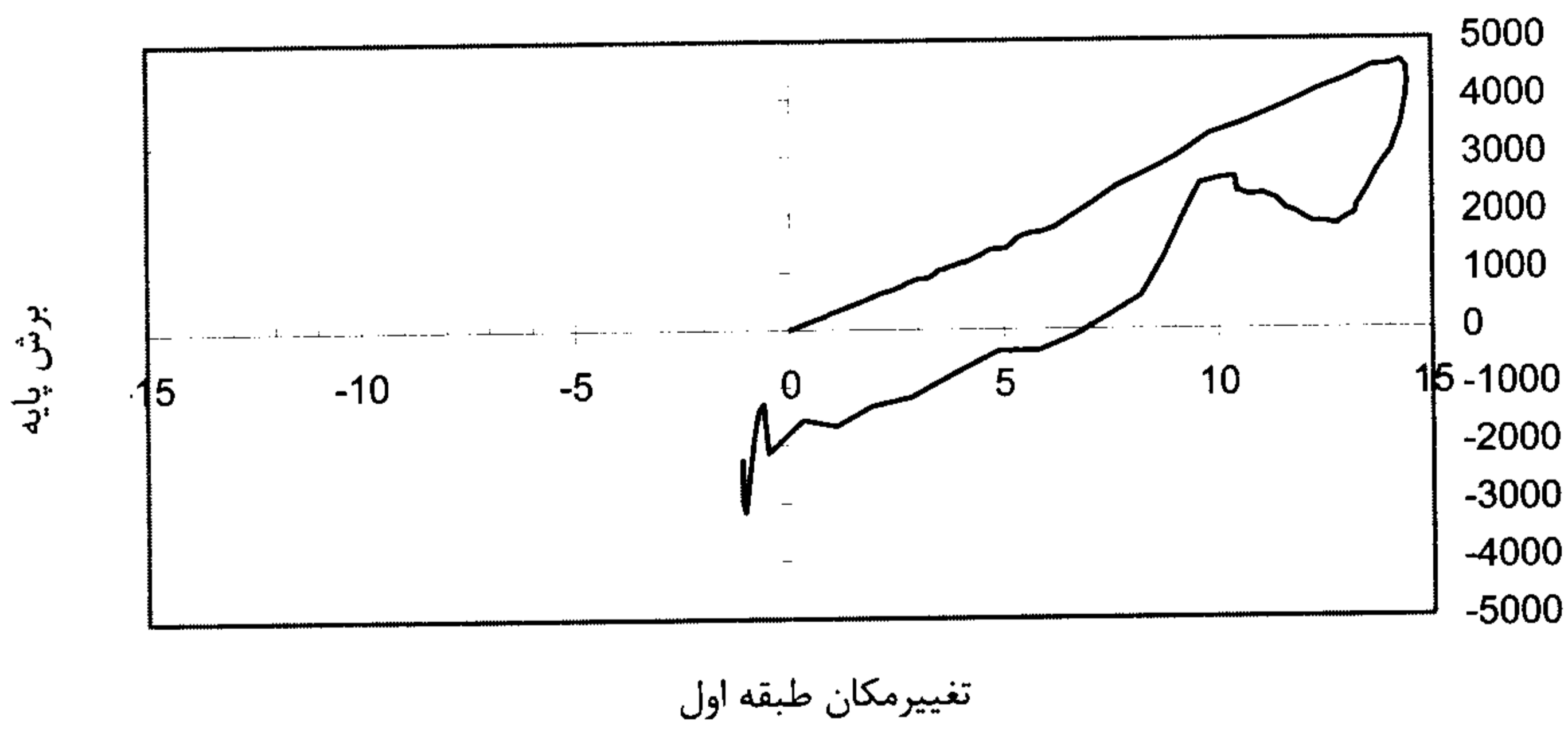
شکل ۱۳: منحنی برش پایه - تغییر مکان افقی طبقه اول قاب خرجینی ساده تحت زلزله ناغان.
