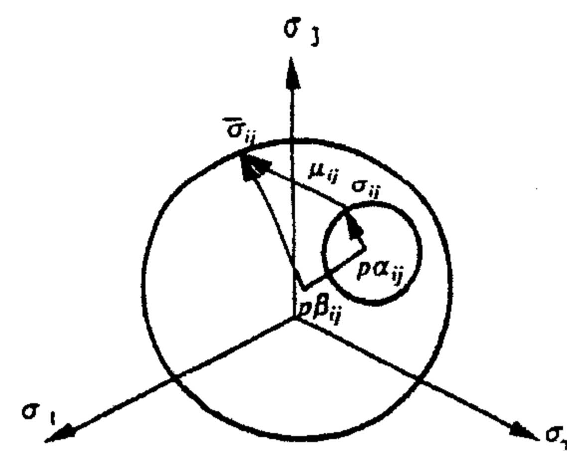
شکل ۱: نمای کلی سطح حدی و سطح تسلیم در فضای تنشهای اصلی.
