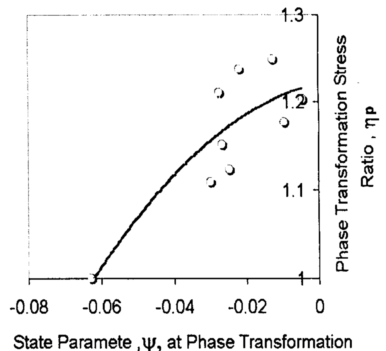
شکل ۵: شیب خط انتقال فاز بر حسب مقدار پارامتر حالت در وضعیت انتقال فاز برای نمونه‌های ساخته شده به روش نمونه‌سازی Wet Tamping (برگرفته از مرجع [۱۵]).
