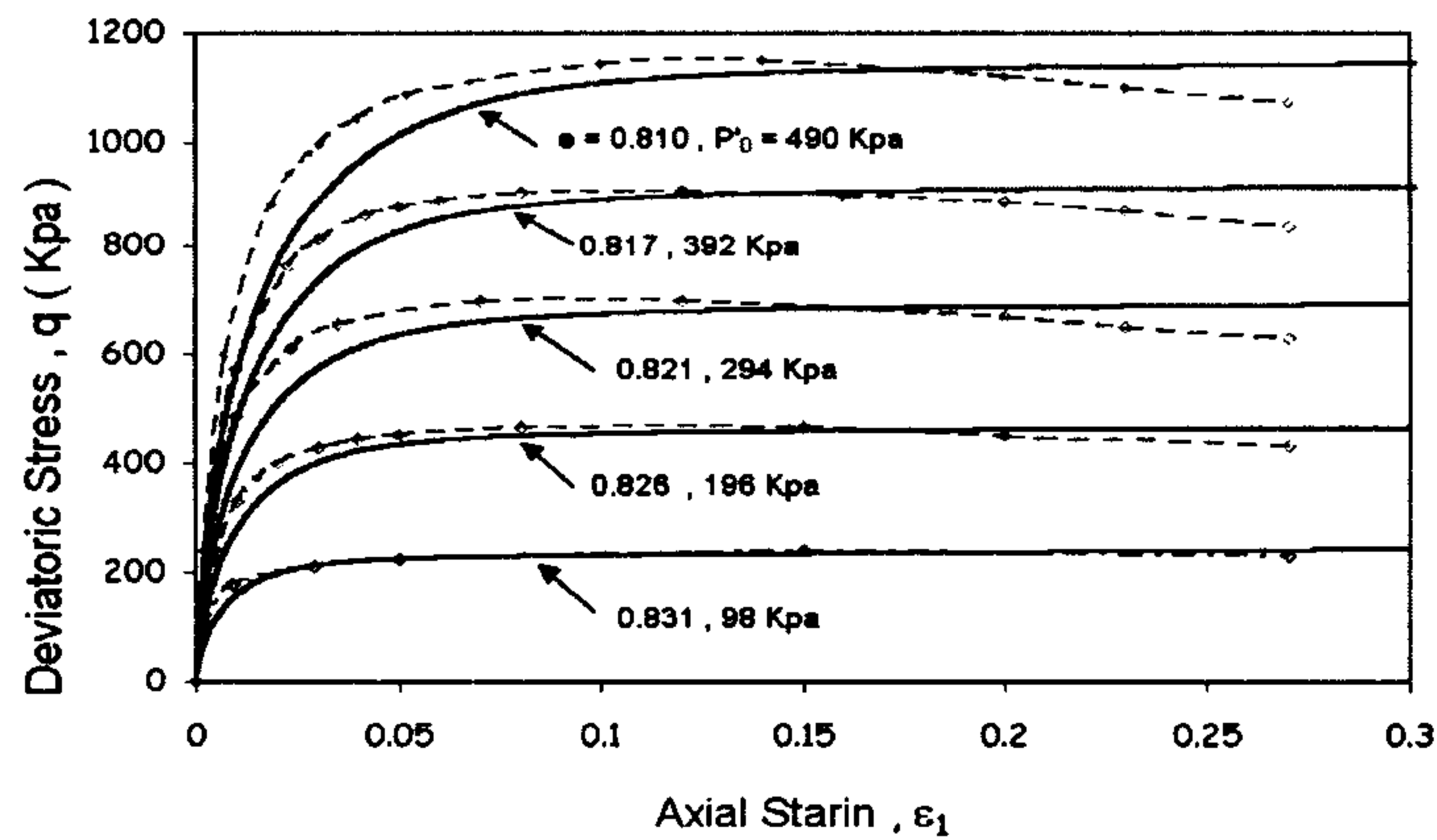
شکل ۱۰: مقایسه نمودارهای تنش - کرنش پیش‌بینی شده توسط مدل اصلاح شده در آزمایشهای سه محوری زهکشی شده با داده‌های تجربی مرجع [۱۵] برای نمونه متراکم ماسه توپورا.
