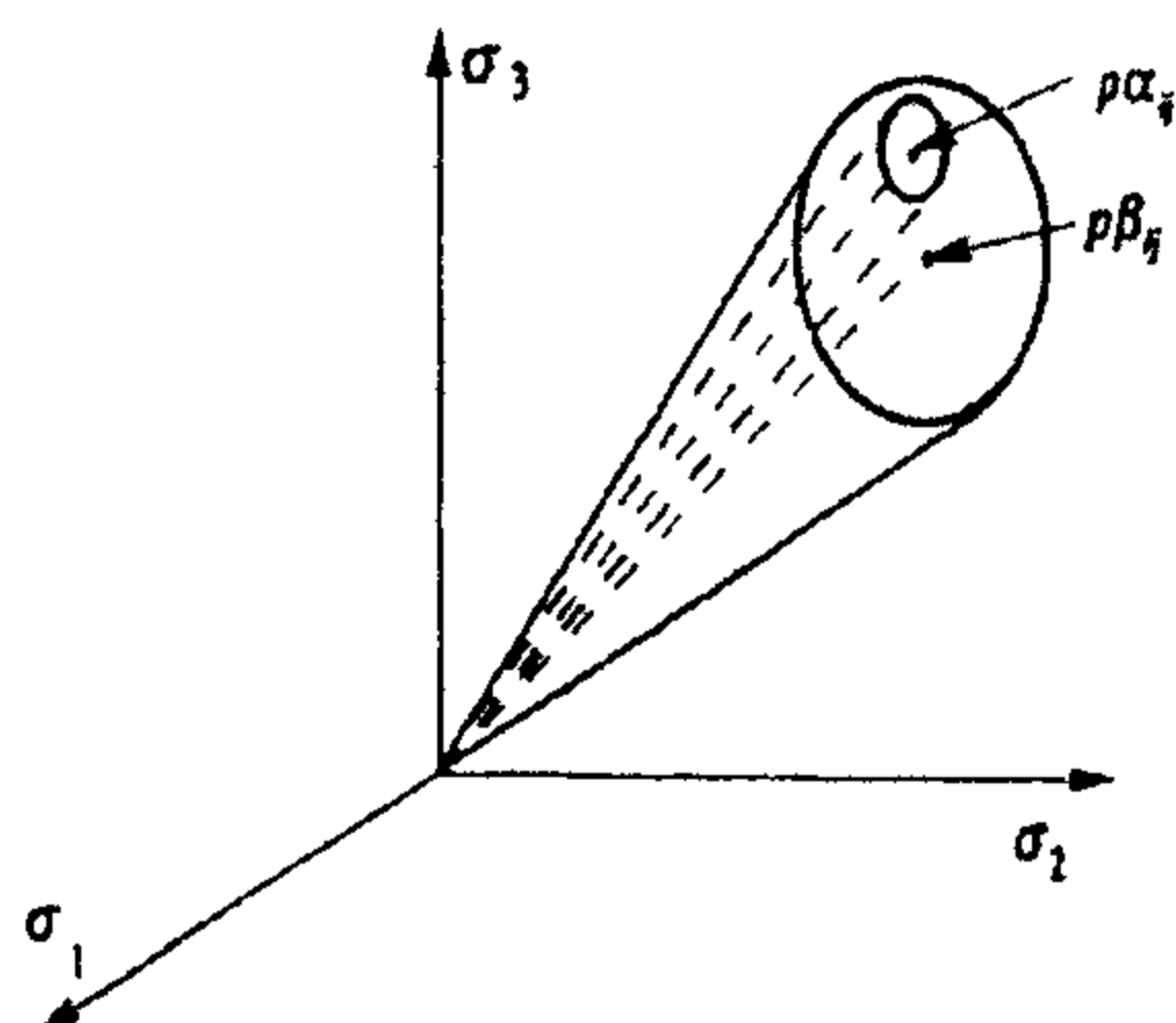
شکل ۲: جابجایی سطح تسلیم در فضای تنشها.
