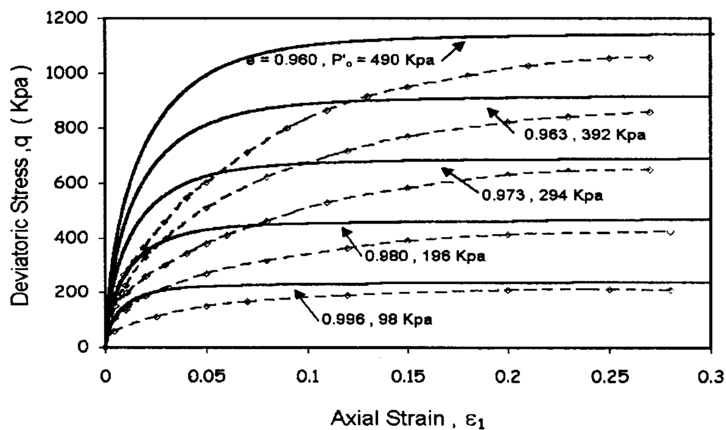
شکل ۱۰: مقایسه نمودارهای تنش - کرنش پیش‌بینی شده توسط مدل اصلاح شده در آزمایشهای سه محوری زهکشی شده با داده‌های تجربی مرجع [۱۵] برای نمونه متراکم ماسه توپورا.
