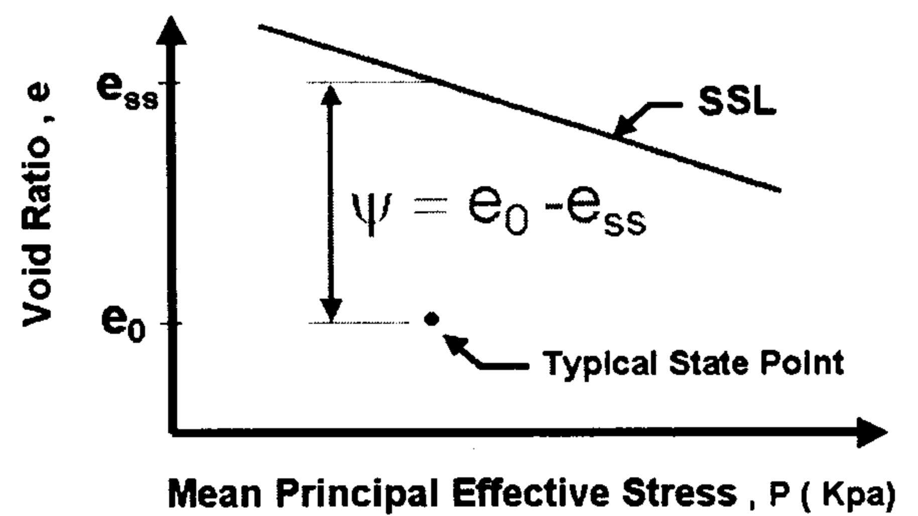
شکل ۴: تعریف پارامتر حالت (بین و جفریز ۱۹۸۵).
