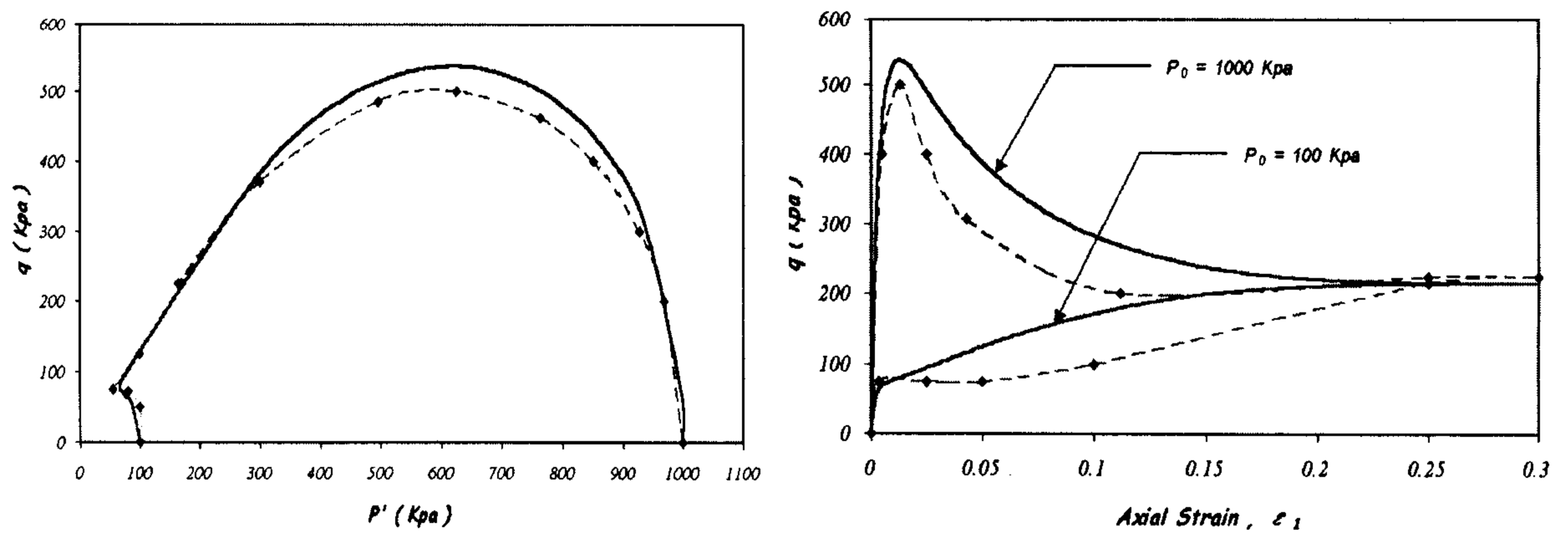
شکل ۸: مقایسه بین نتایج پیش بینی مدل اصلاح شده با داده های تجربی مرجع [۱۵] برای ماسه توپورا ( e = 0.907 ) در بارگذاری زهکشی نشده.
