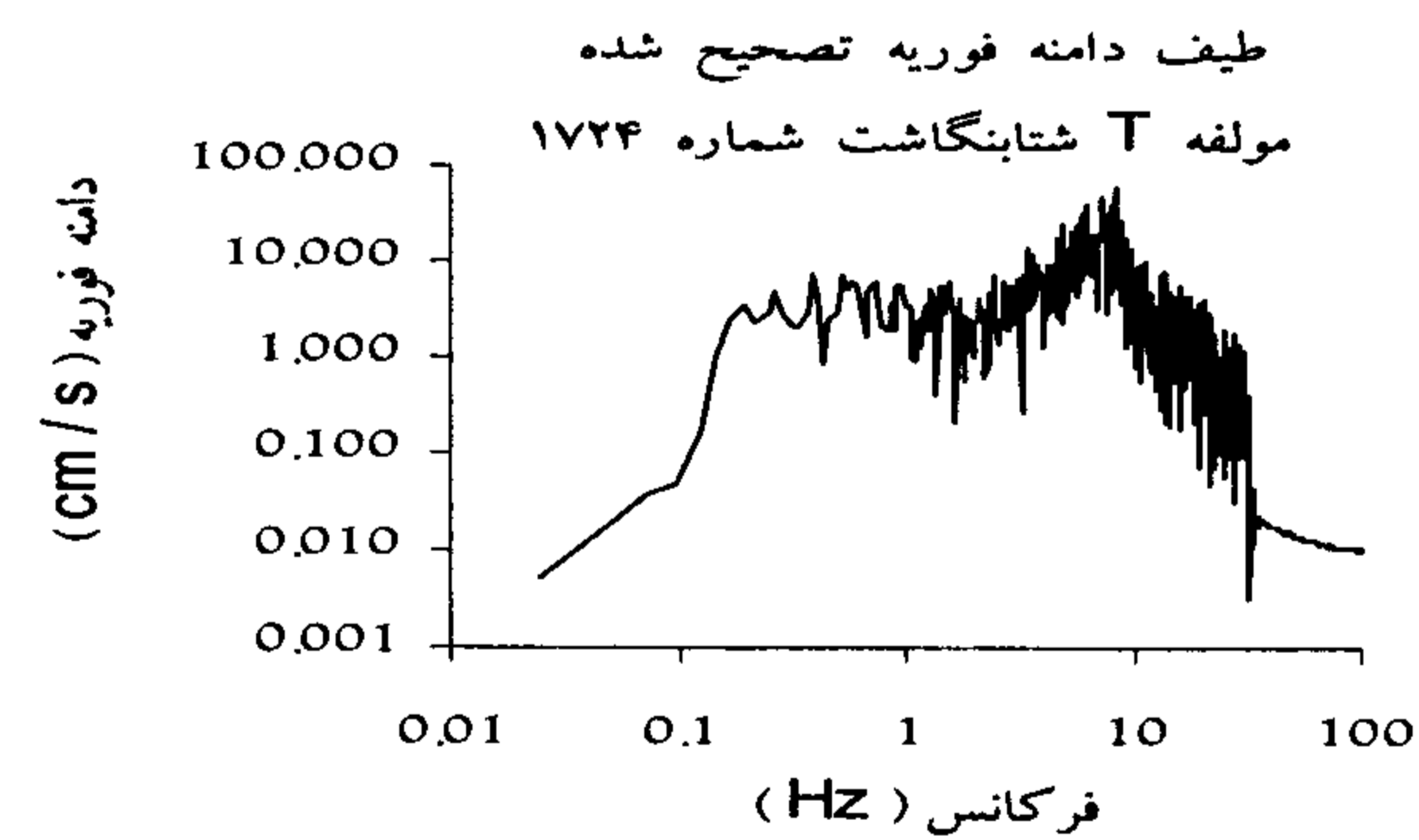
شکل ۷: طیف دامنه فوریه زمین لرزه ای با بزرگای زیاد.
