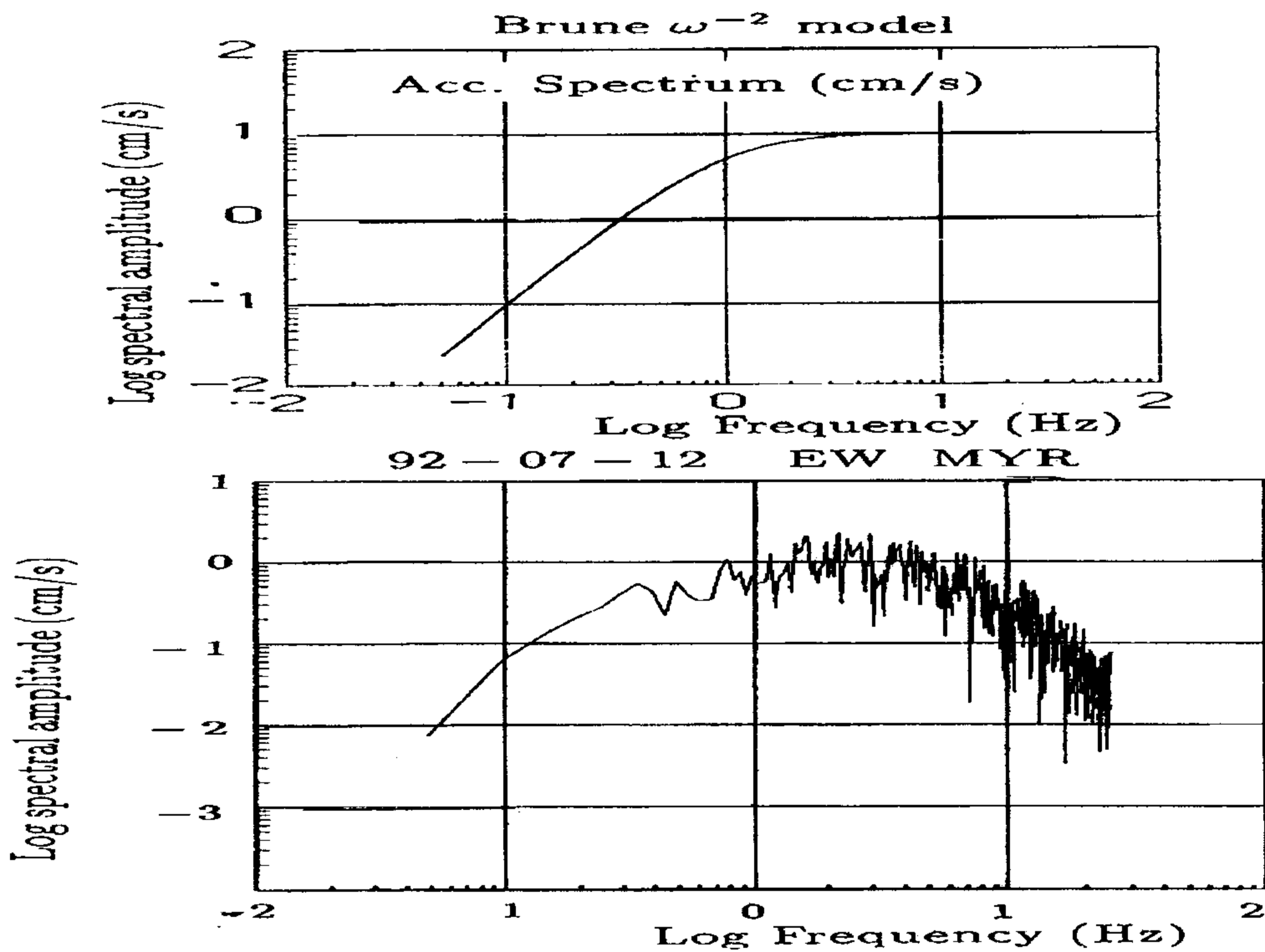
شکل ۶: مقایسه طیف دامنه فوریه شتاب زمین لرزه ۱۲ ژولای ۱۹۹۲ زاین ثبت شده
