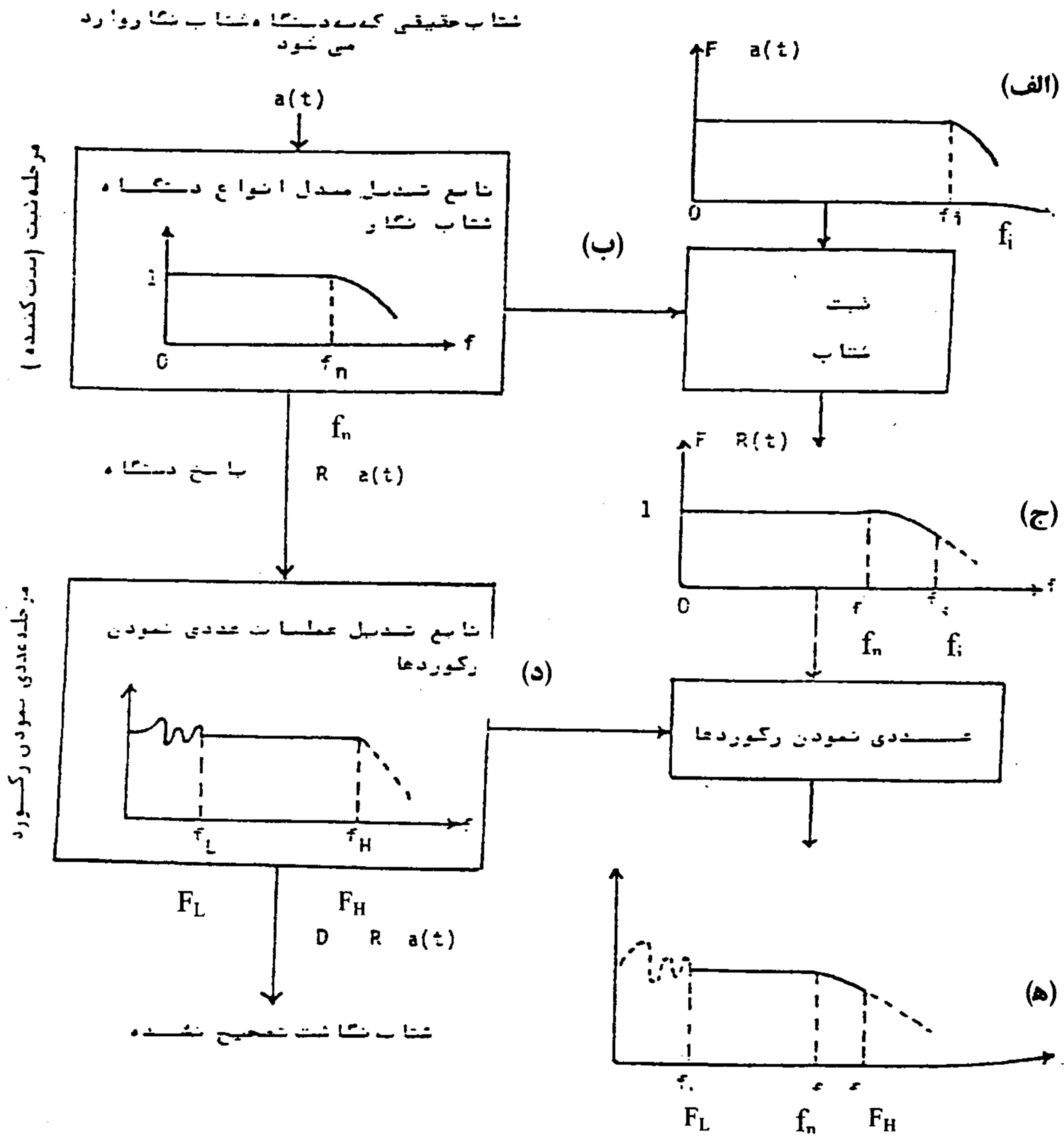
شکل ۱: تغییرات کتاب در مراحل ثبت و عددی نمودن آن [۴].
