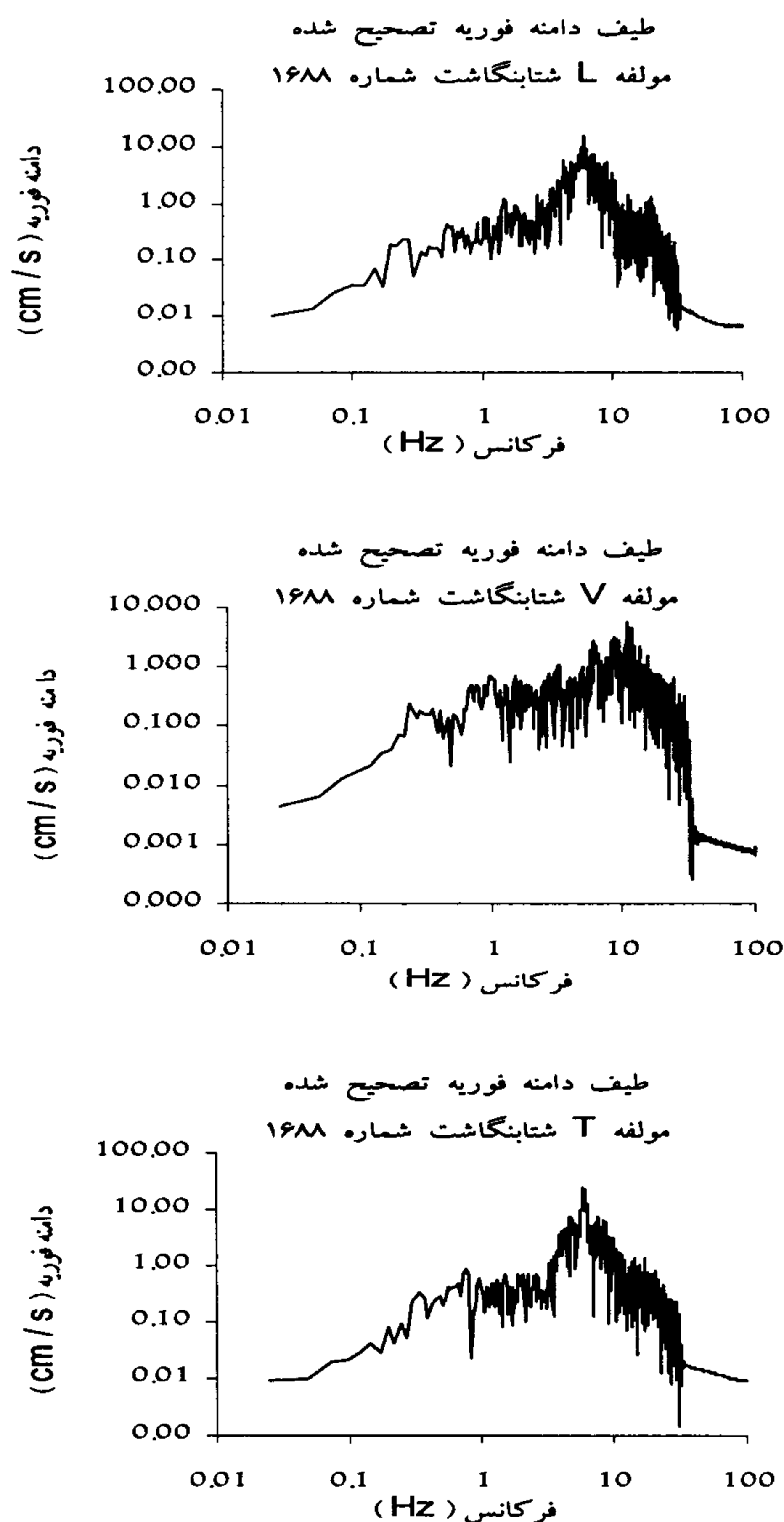
شکل ۸: طیف دامنه فوریه زمین لرزه ای با بزرگای کم.
