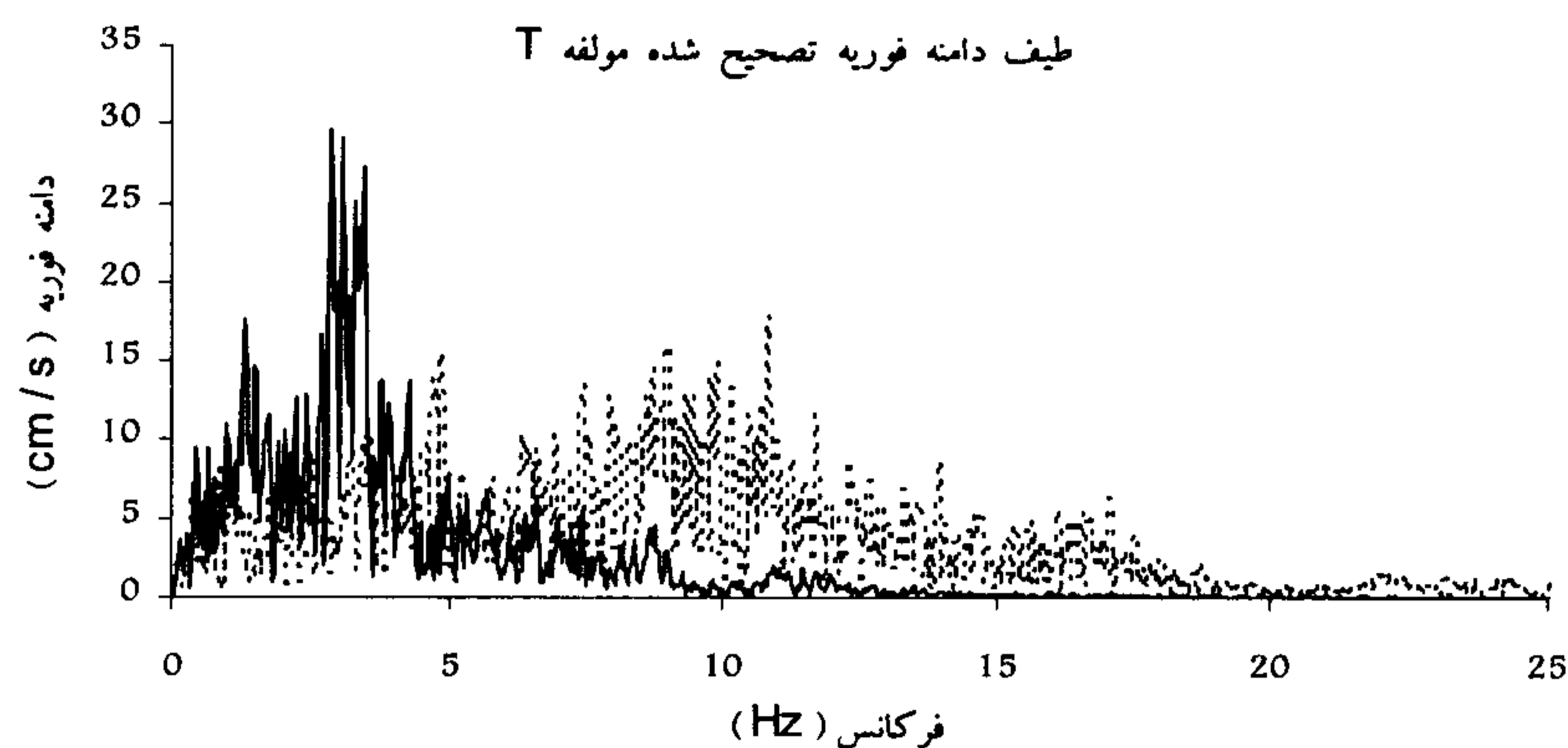
شکل ۹: مقایسه محتوای فرکانسی شتاب ثبت شده یک زمین لرزه در شرایط مختلف ساختمانی.
