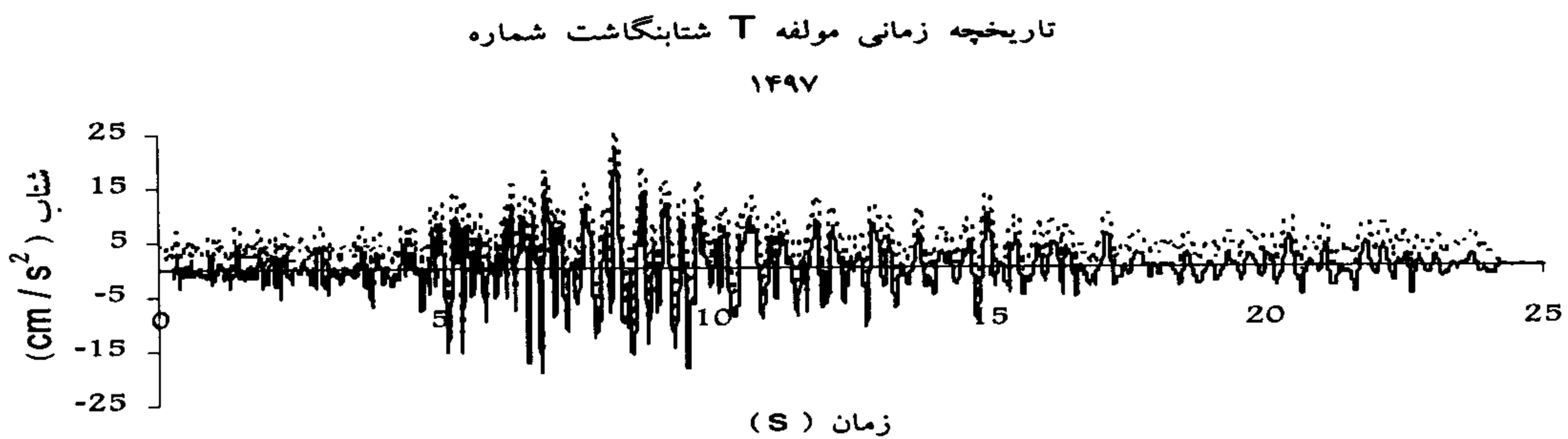
شکل ۴: اثر تصحیح خط مبنا بر تاریخچه زمانی شتاب.
