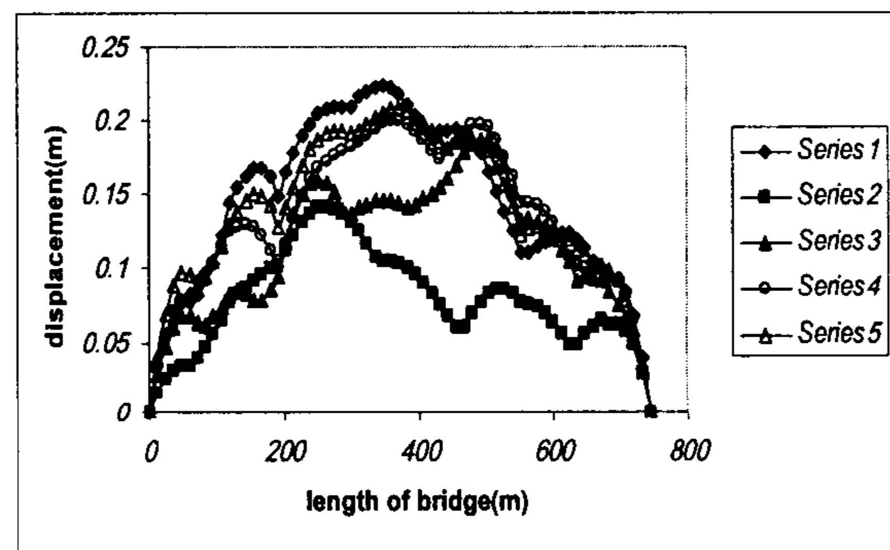
شکل ۳۴: تغییر مکان طولی ماکزیمم عرشه پل شماره ۳ در اثر تحریک هماهنگ (series1) و ناهماهنگ و با تاخیر زمان در تکیه گاهها (series2 تا series5).
