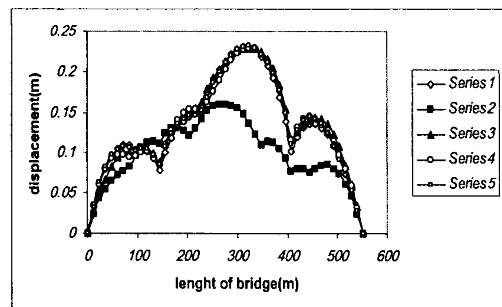
شکل ۲۷: تغییر مکان طولی ماکزیمم عرشه پل شماره ۲ در اثر تحریک هماهنگ (series1) و ناهماهنگ تکیه گاهها (series2 تا series5).
