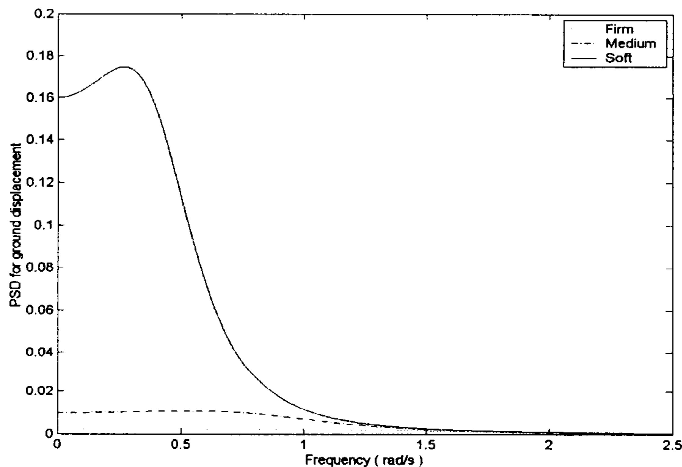
شکل ۲۰: نمودار تابع چگالی طیف توان بر حسب فرکانس برای سه نوع خاک نرم و متوسط و سخت.
