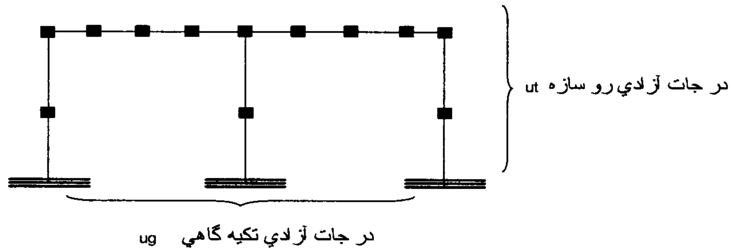
شکل ۱۹: تعریف درجات آزادی روسازه و تکیه گاه ها.
