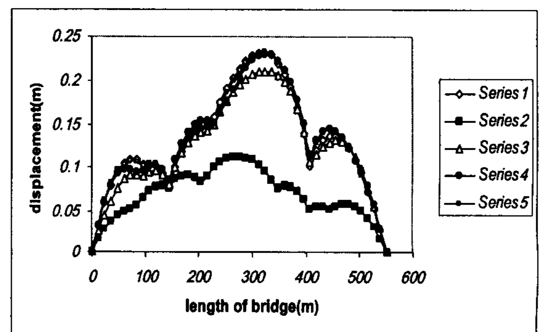
شکل ۳۳: تغییر مکان طولی ماکزیمم عرشه پل شماره ۲ در اثر تحریک هماهنگ (series1) و ناهماهنگ و با تاخیر زمان در تکیه گاهها ( series2 تا series5 ).
