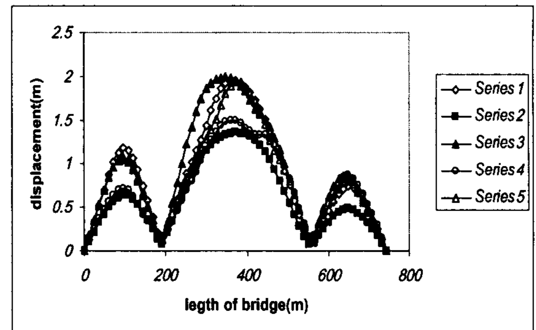
شکل ۴۰: تغییر مکان عرضی ماکزیمم عرشه پل شماره ۳ در اثر تحریک هم‌هنگ (series1) و با تاخیر زمان در تکیه گاهها ( series2 تا series5 ).
