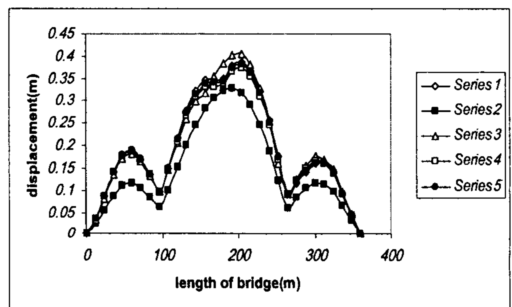
شکل ۴۱: تغییر مکان عرضی ماکزیمم عرشه پل شماره ۱ در اثر تحریک هم‌هنگ (series1) و ناهماهنگ و با تاخیر زمان در تکیه گاهها ( series2 تا series5 ).
