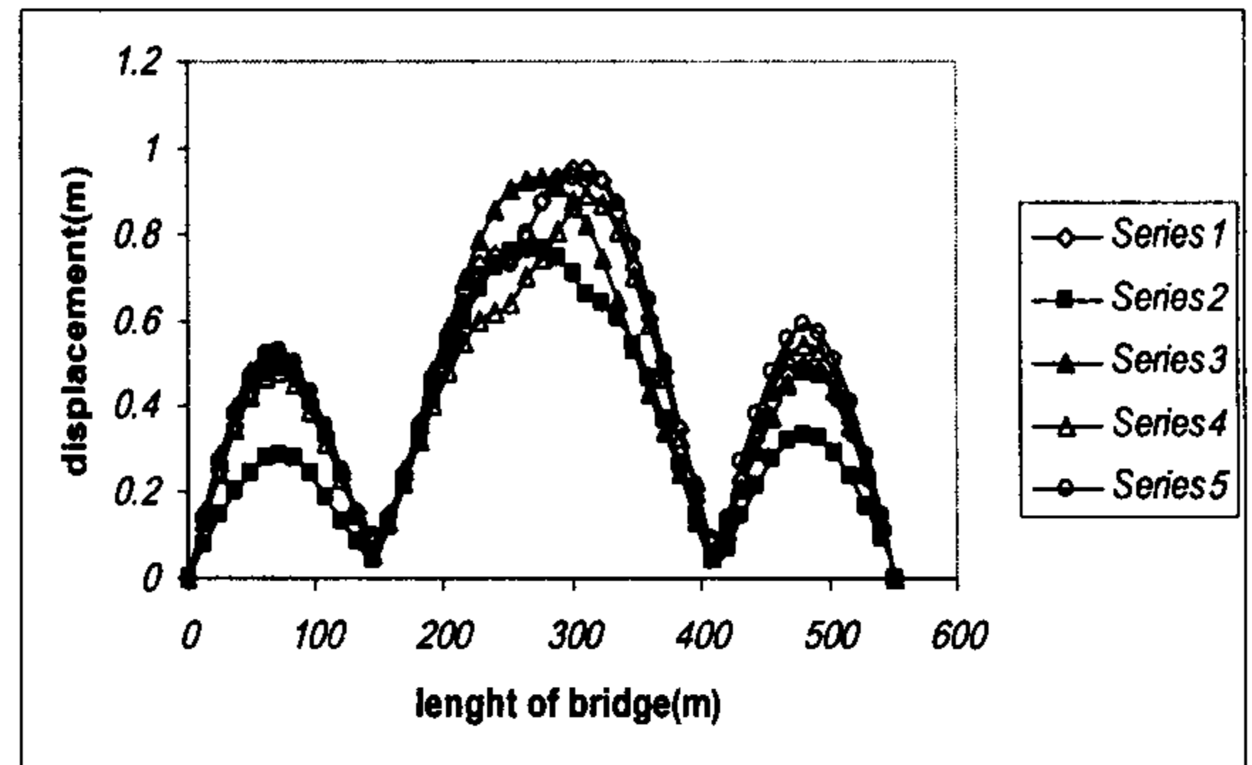
شکل ۳۹: تغییر مکان عرضی ماکزیمم عرشه پل شماره ۲ در اثر تحریک هم‌هنگ (series1) و با تاخیر زمان در تکیه گاهها ( series2 تا series5 ).
