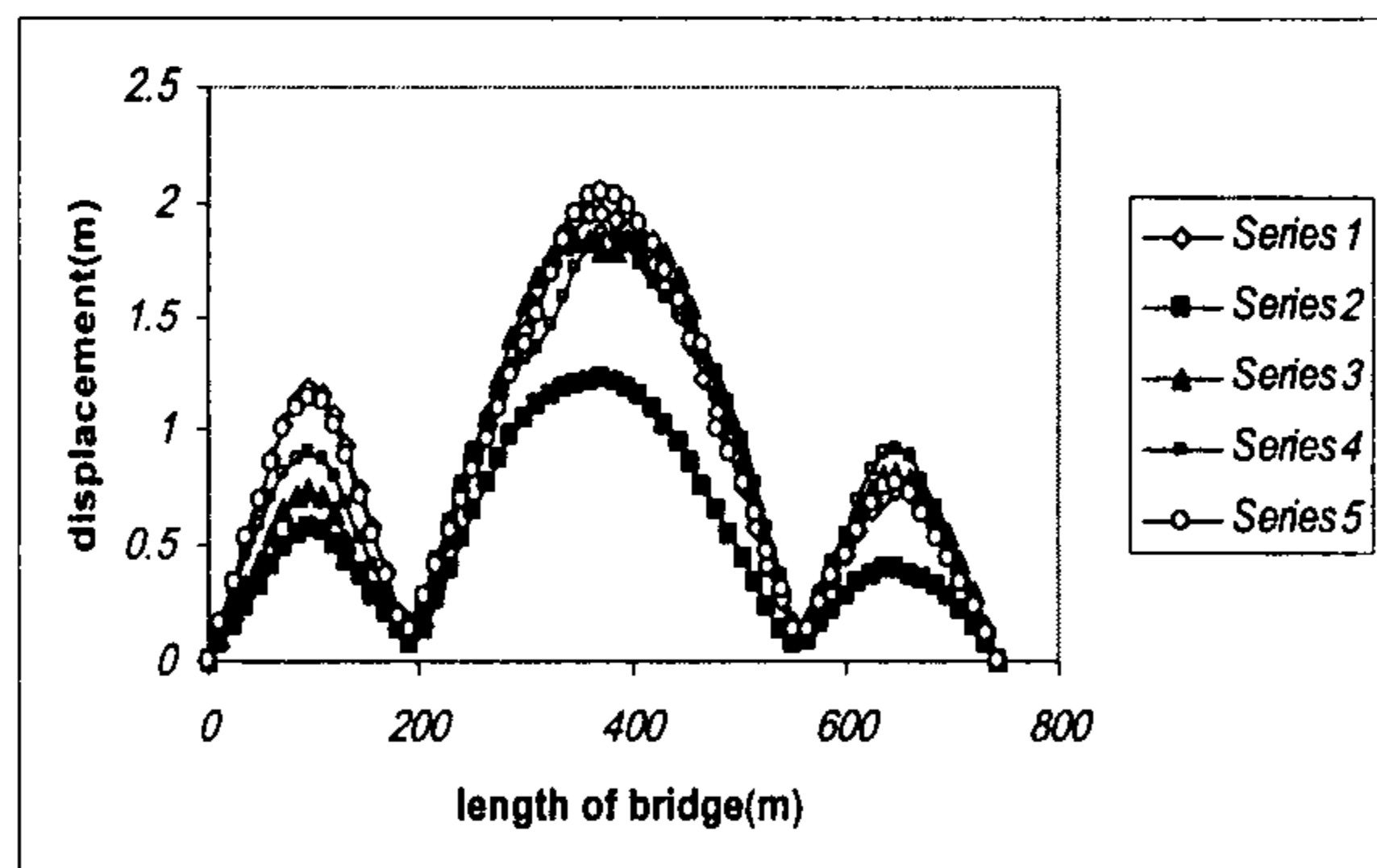
شکل ۴۳: تغییر مکان عرضی ماکزیمم عرشه پل شماره ۳ در اثر تحریک هم‌هنگ (series1) و ناهماهنگ و با تاخیر زمان در تکیه گاهها ( series2 تا series5 ).
