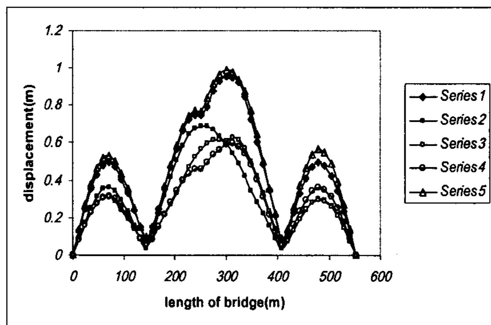
شکل ۴۲: تغییر مکان عرضی ماکزیمم عرشه پل شماره ۲ در اثر تحریک هم‌هنگ (series1) و ناهماهنگ و با تاخیر زمان در تکیه گاهها ( series2 تا series5 ).
