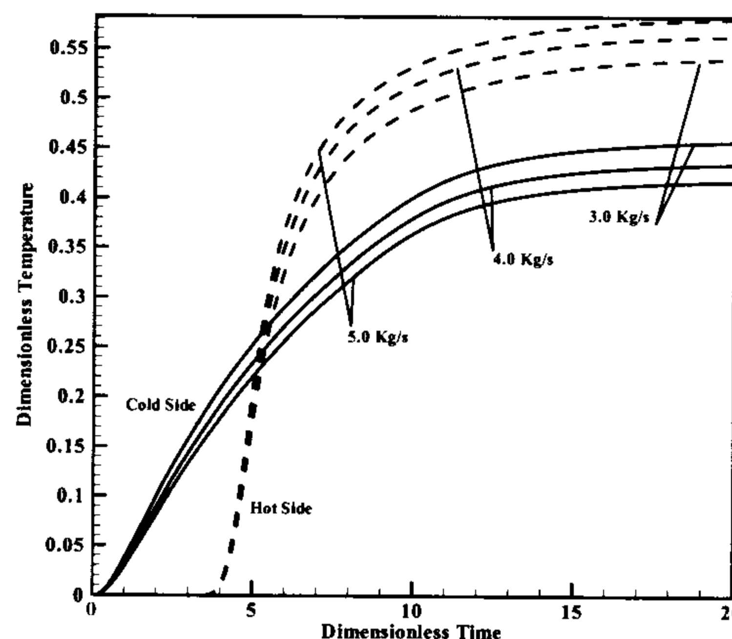
شکل ۸: درجه حرارت حالت گذرای مبدل حرارتی U دارای 10 کانال، مدل متغیر، (- -) سمت گرم، (-) سمت سرد دبی ورودی: 3.0، 4.0، 5.0 kg/s، بازدهی به ترتیب: 45.8%، 43.6% و 41.8%.
