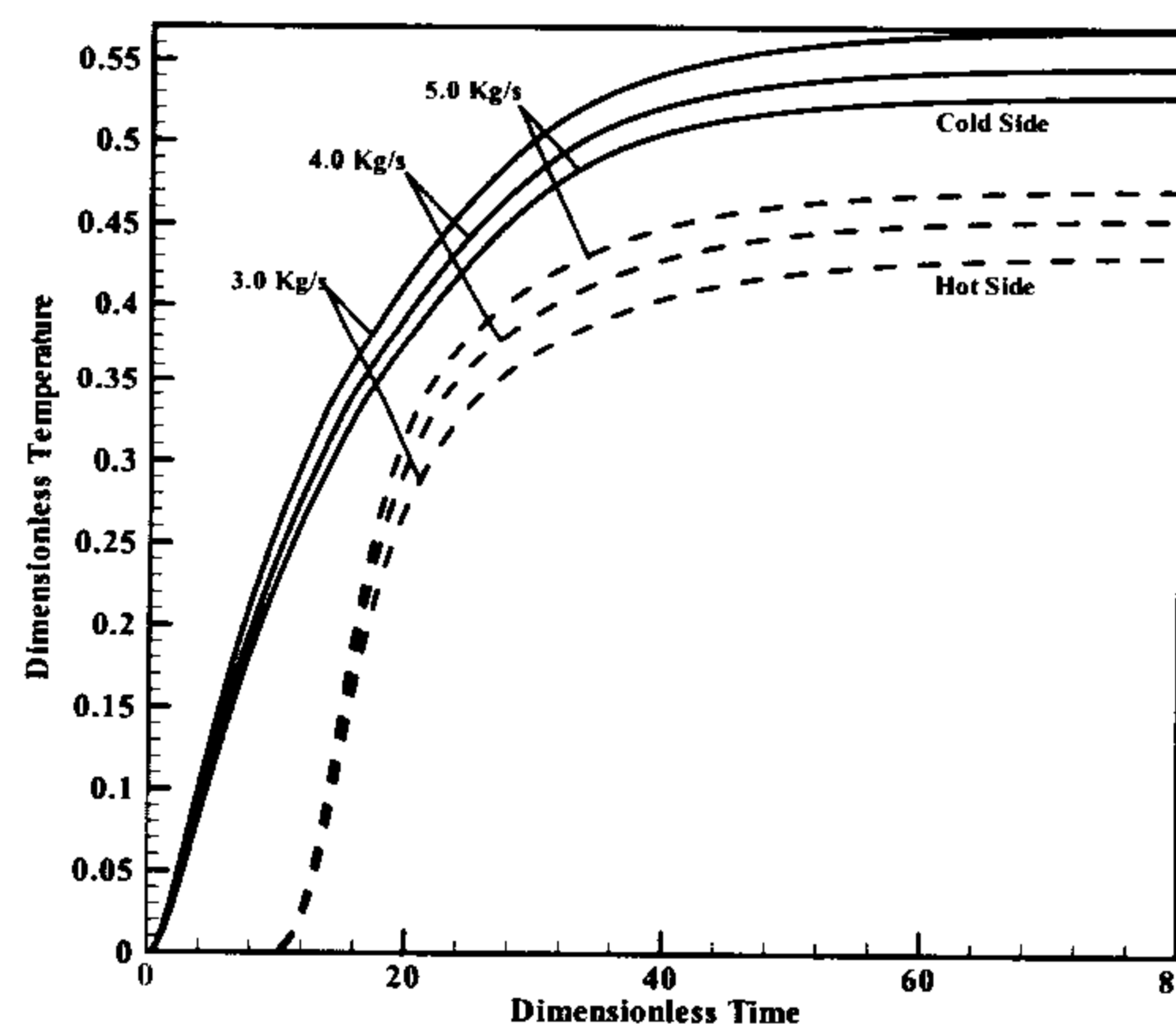
شکل ۹: درجه حرارت حالت گذرای مبدل حرارتی U دارای 30 کانال، مدل متغیر، (- -) سمت گرم، (-) سمت سرد دبی ورودی: 3.0، 4.0، 5.0 kg/s، بازدهی به ترتیب برابر 56.8%، 55.0% و 53.0%.
